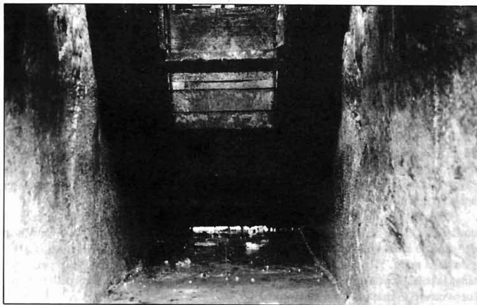
FIGURA 12. Solera de la acequia debajo de la noria, limpia de materiales gruesos y con una pendiente importante.
