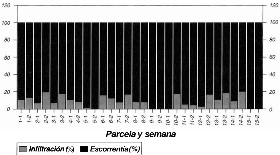
FIGURA 4. Porcentajes de infiltración. En todos los casos son muy elevados debido al déficit hídrico que presenta el suelo al principio de las pruebas.
