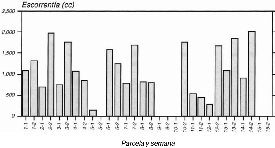
FIGURA 3. Comportamiento de la escorrentía durante la experiencia. En general, la respuesta hídrica es mayor durante la segunda prueba.
