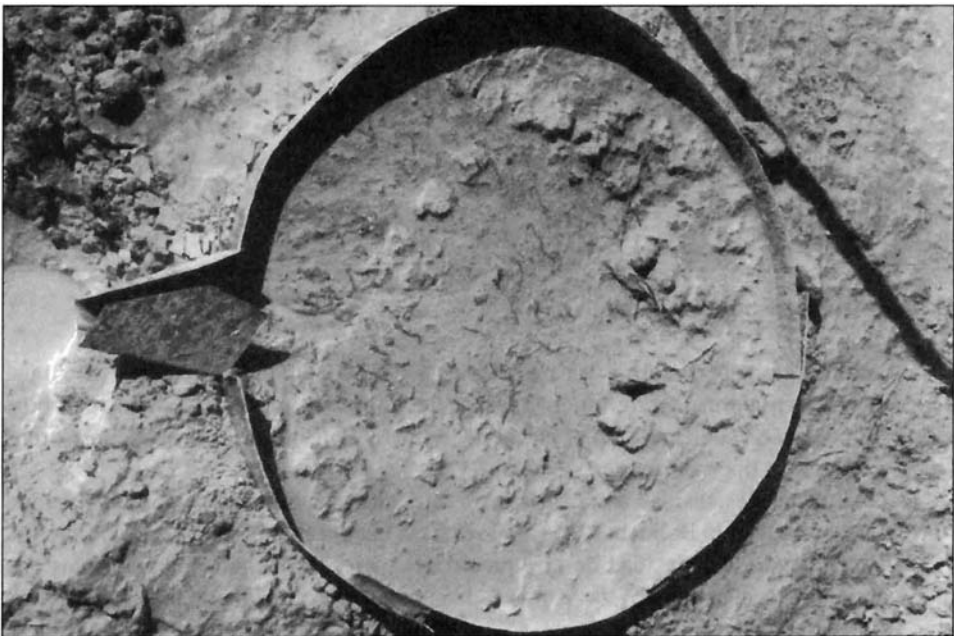
FIGURA 6. Aspecto de la morfología superficial de un suelo margoso de badland por impacto de las gotas de lluvia y la escorrentía superficial, tras un experimento de 30 minutos de lluvia, con intensidad de 55 \text{ mm}\cdot\text{h}^{-1} y sobre microparcela circular de 0,25 \text{ m}^2 .
