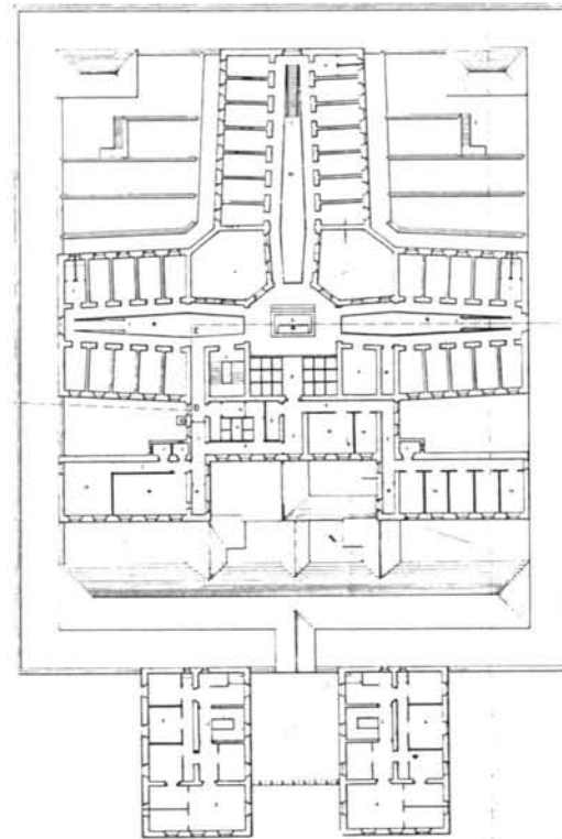
Lámina 3. Proyecto de Cárcel de Audiencia.
