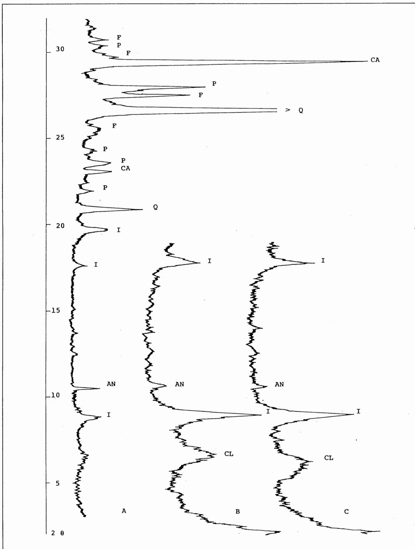
Fig. 3. Difractogramas de la muestra n.º 6. A: Polvo, B: Agregado orientado, C: Agregado orientado tratado con etilenglicol, Q: Cuarzo, CA: Calcita, P: Plagioclasas, F: Feldespatos, I: Ilita, CL: Clorita, AN: Anfíboles.
