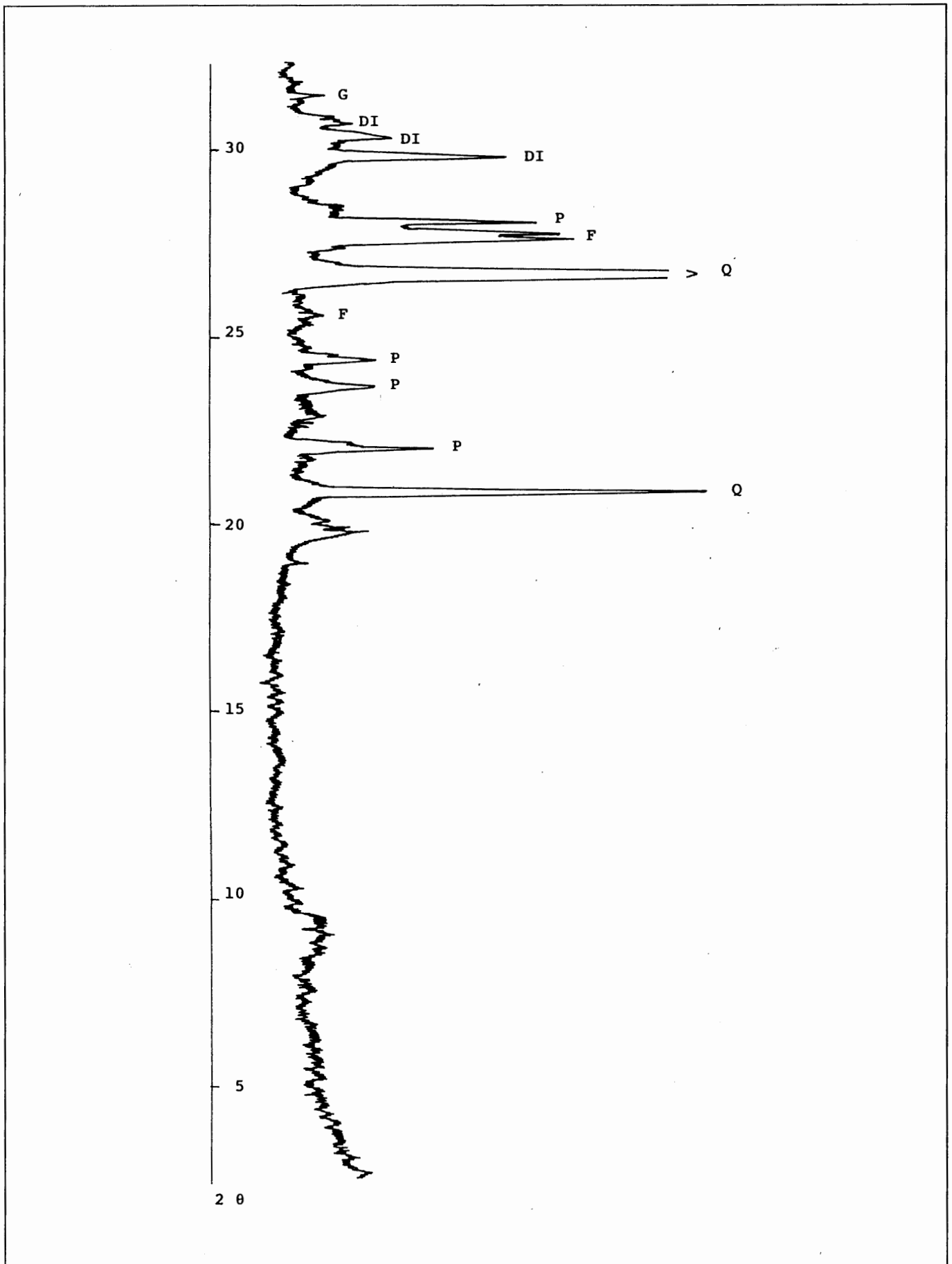
Fig. 5. Difractograma de la muestra n.º 8. Q: Cuarzo, P: Plagioclasas, F: Feldespatos, DI: Diópsido, G: Gehlenita.
