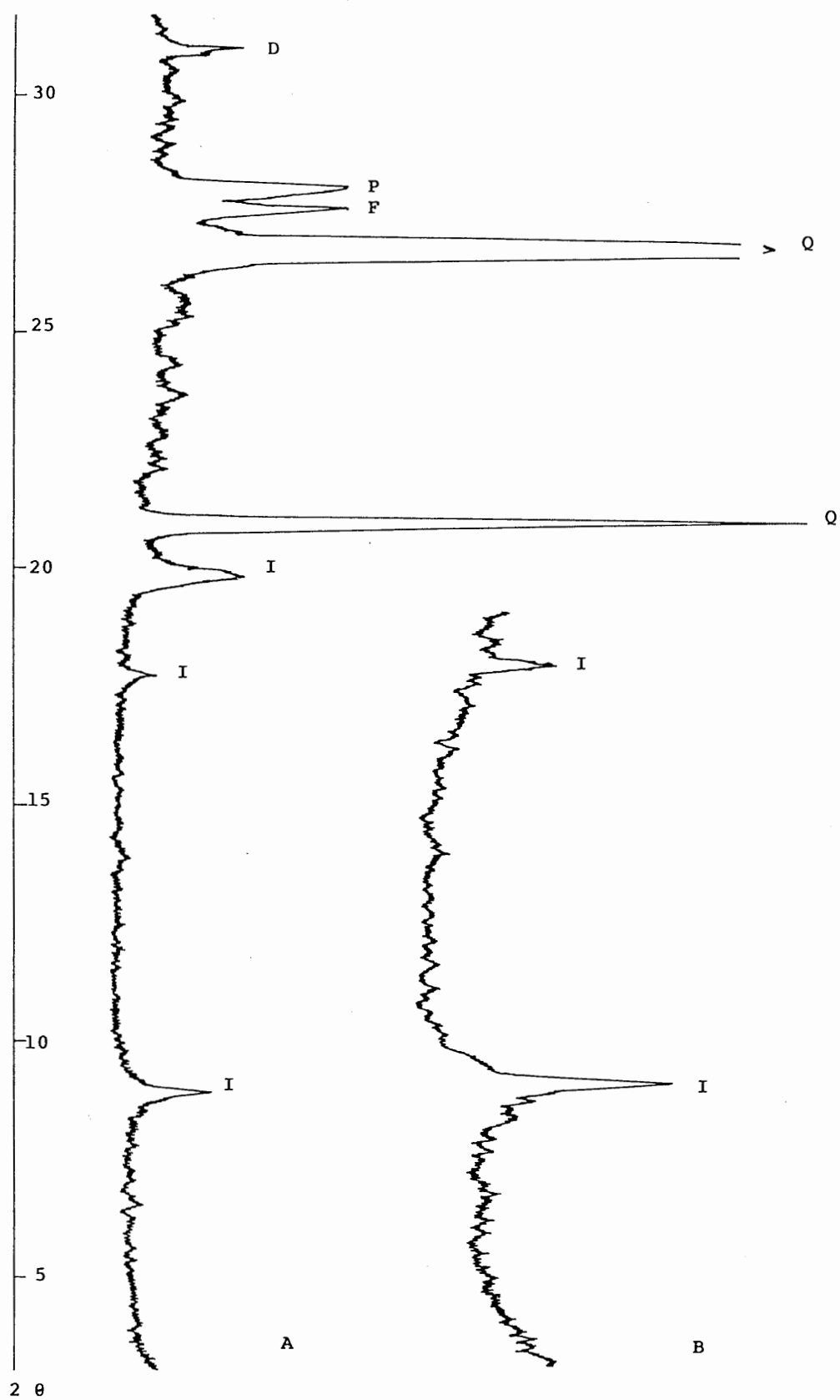
Fig. 4. Difractogramas de la muestra n.º 7.
