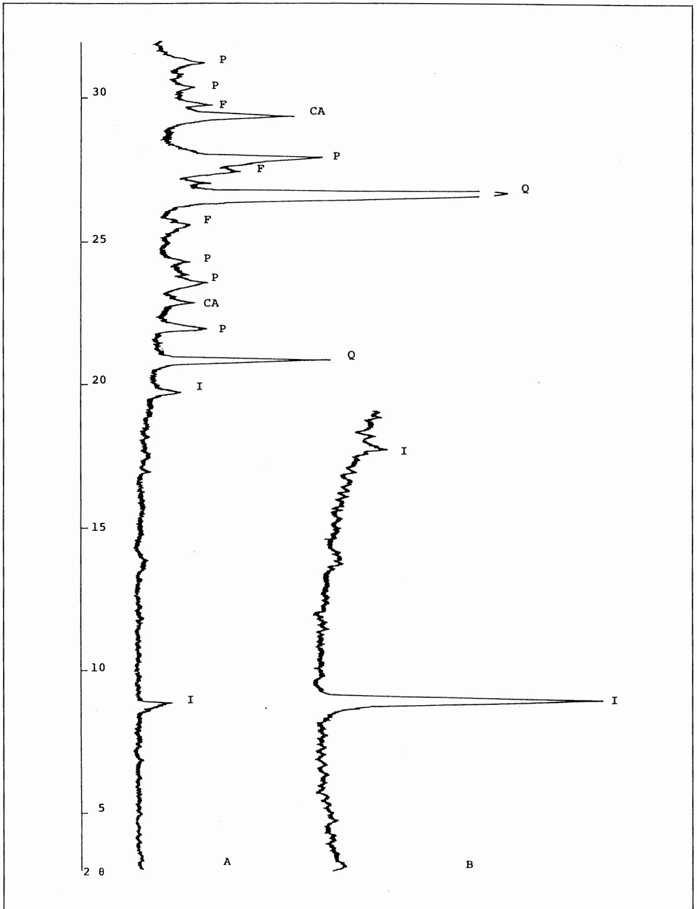
Fig. 1. Difractogramas de la muestra n.º 4.
