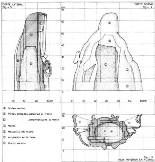
Figura 3. Vista Inferior en Planta.
