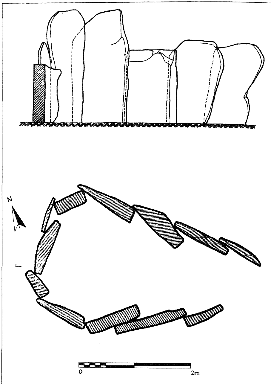
Figura 5. Monte Pirleo 2, planta e sección da cámara, segundo o informe inédito.
