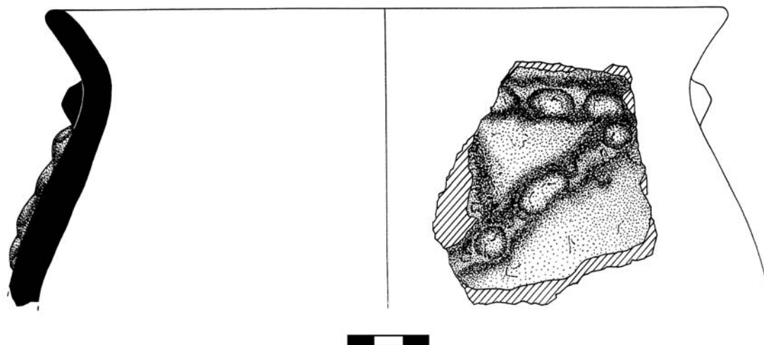
Figura 5. Vasija de grandes dimensiones con decoraciones plásticas. Diámetro real de la boca: 25'03 cm. Cabezo Chinchón. Dibujo: Héctor Arcusa Magallón.
