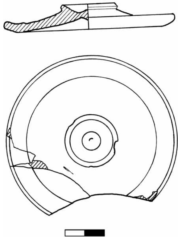
Figura 26. Tapadera de la forma 7 hispánica que cubría la olla. Dibujo: Héctor Arcusa Magallón.
