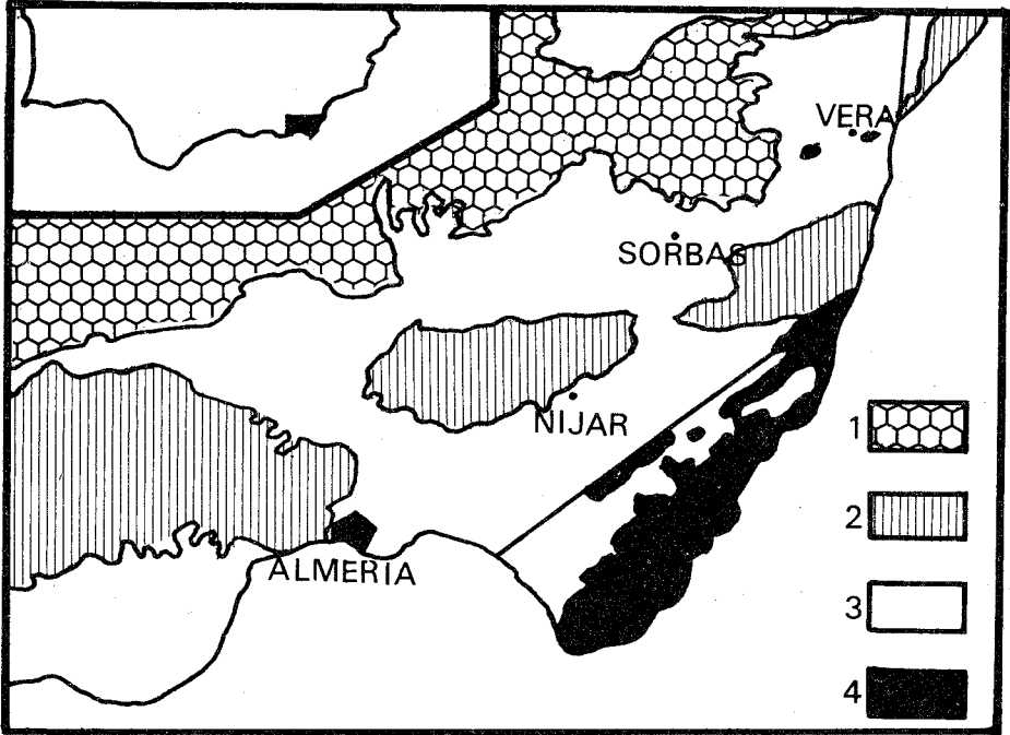
Fig. 1. Situación Geológica y Geográfica del área de estudio. 1. Complejo Nevado-Filábride. 2. Complejo Alpujarride. 3. Materiales sedimentarios Postorogénicos. 4. Materiales volcánicos.
