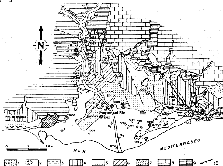
Figura nº 2. Plano hidrogeológico del delta del río Adra. 1 a 7 materiales neógeno-cuaternarios (1: conos de deyección; 2: marismas; aluviales y delta actual; 3: limos rojos; 4: glacis; 5: glacis cementado; 6: conglomerados "facies deltaica"; 7: calcarenitas; 8 y 9: materiales alpujárrides (8: calizas y dolomías; 9: esquistos, filitas y cuarcitas) 10: manto de corrimiento.
