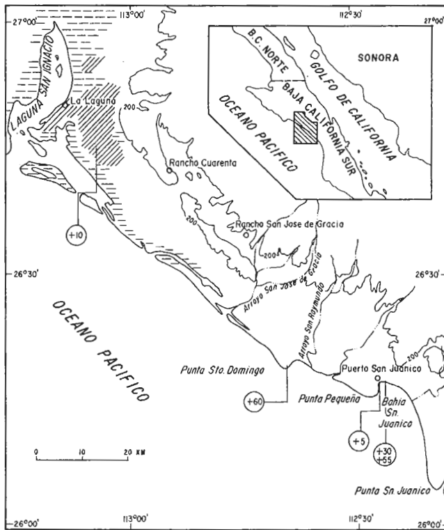
Figura 12.—Mapa de localización de las terrazas marinas pleistocénicas observadas entre los paralelos 26° y 27° N en la costa del Pacífico. Las alturas están indicadas en metros sobre el nivel medio del mar.
