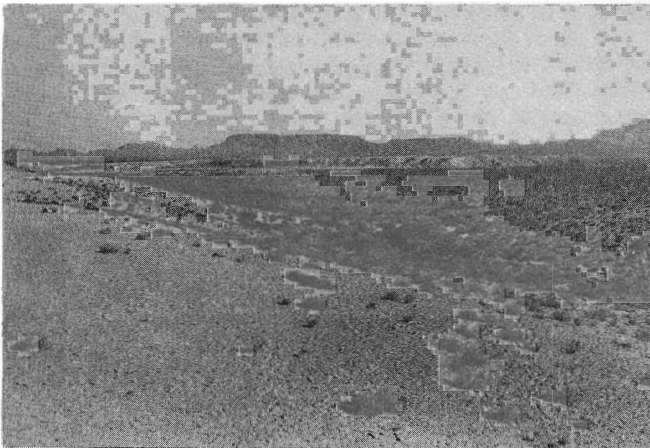
Figura 4.—Aspecto de la coquina con Tivela stultorum , al norte de La Bocana. Estos depósitos litorales, constituidos por arenas y fragmentos muy abundantes de conchas de Tivela stultorum (visibles en el primer plano), tienen una gran extensión lateral. La coquina tiene un espesor de varios metros y alcanza alturas máximas de + 20 m.
