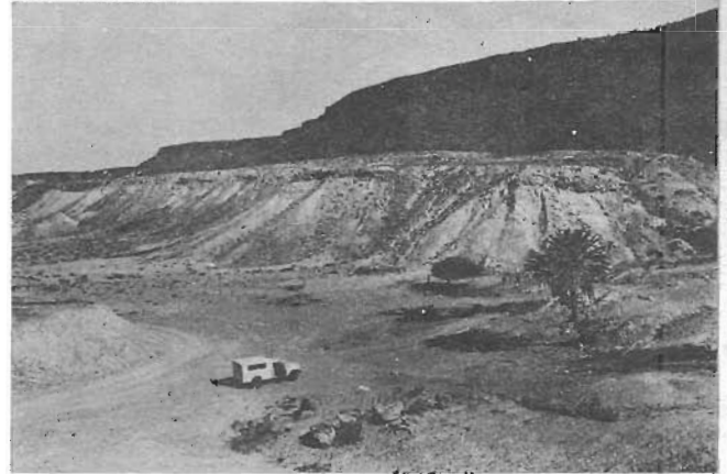
Figura 13.—Terraza marina del Pleistoceno temprano en Puerto San Juanico. Areniscas conglomeráticas y fosilíferas cubren, en el segundo plano, un depósito pliocénico erosionado subhorizontalmente. Esta capa de areniscas, de espesor inferior a 5 m, yace a + 30 m de altura. En el fondo, derrames basálticos descansan sobre los mismos depósitos pliocénicos que son visibles en el centro.
