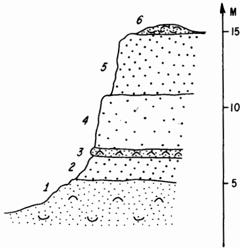
Figura 9.—Sección que muestra depósitos infrayaciendo a la coquina con Tivela stultorum , 10 km al sur del arroyo San Rafael, (1) Areniscas gris verdáceas con moldes de conchas (Plioceno?); (2) arenas verdes (Plioceno?); (3) arenas y areniscas gris claras, fosilíferas (Pleistoceno inferior o medio?); (4) arenas eólicas rojizas; (5) arenas eólicas de color crema; (6) depósito alterado y encalichado, con numerosas Tivela stultorum .
