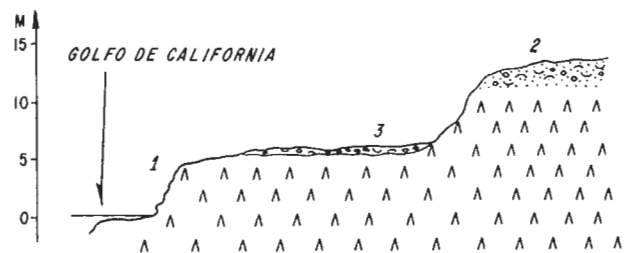
Figura 18.—Sección de las terrazas marinas pleistocénicas en la costa de la Misión de San Bruno, a 20 km al norponiente de Loreto. (1) Zócalo volcánico (Mioceno); (2) depósito marino encañado (Pleistoceno temprano o mediano); (3) depósito marino más reciente (Sangamoniano ?).
