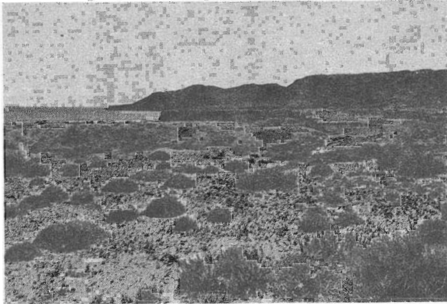
Figura 6.—Terraza de abrasión en Punta Quebrada. En el primer plano, arenas y conchas retrabajadas. En el segundo plano, así como en la punta en el fondo, se distingue la forma característica de las terrazas marinas. Depósitos litorales, de unos decímetros de espesor, cubren una plataforma de abrasión marina. La superficie de las plataformas está a + 5 m de altura.
