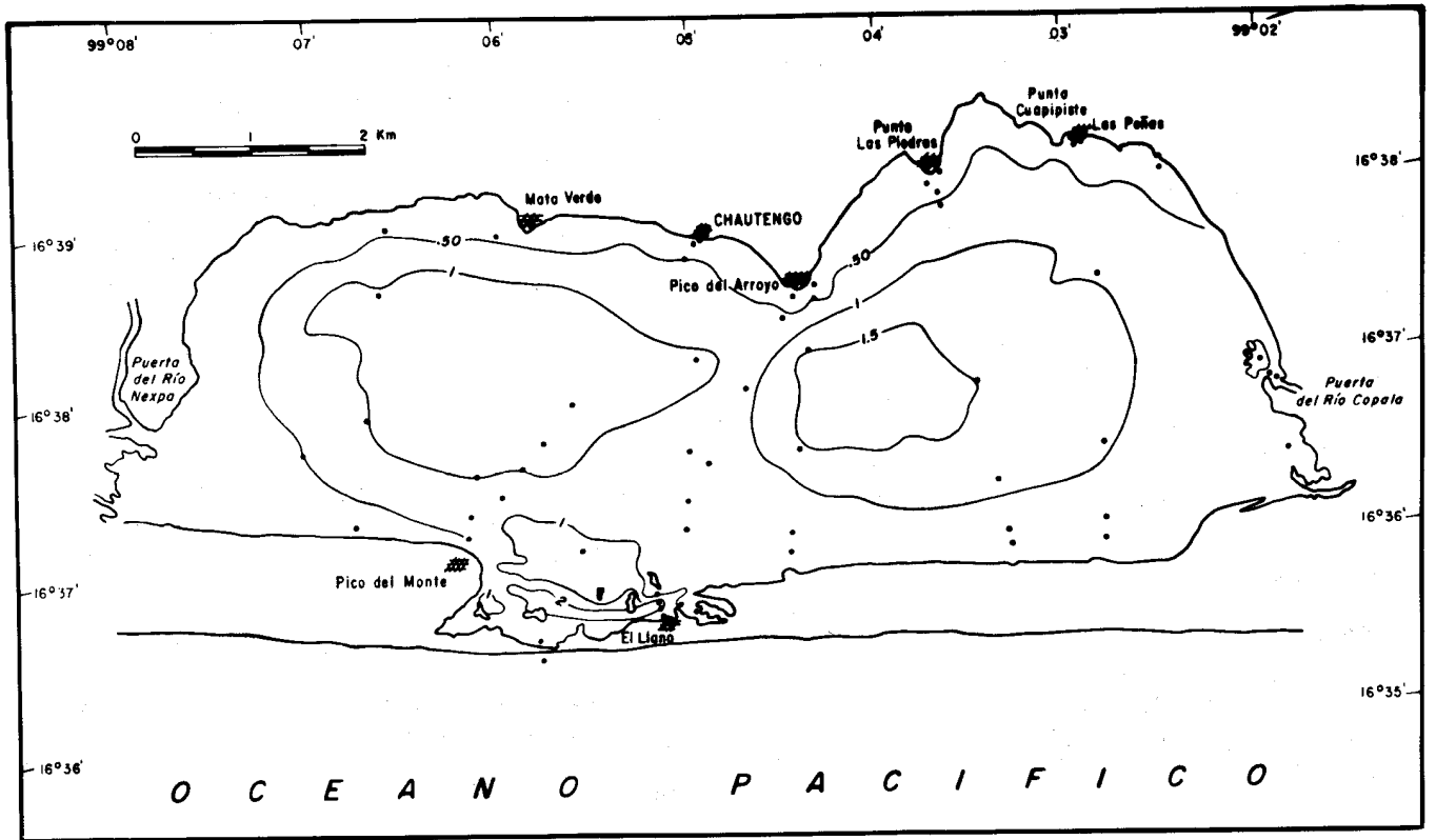
Figura 2.- Batimetría de la laguna. Isóbatas en metros.
