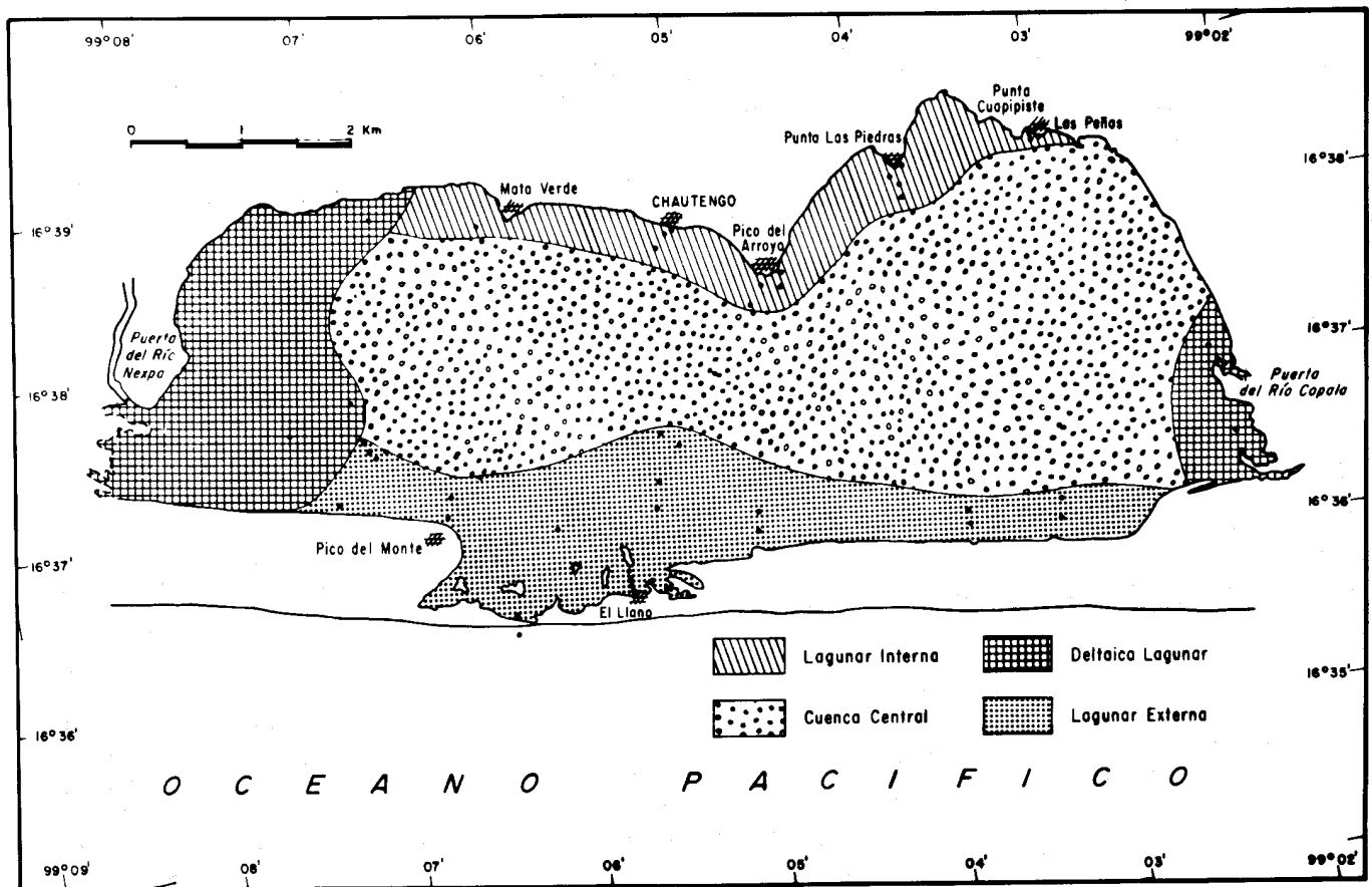
Figura 11.- Areas faunísticas en la Laguna de Chautengo.
