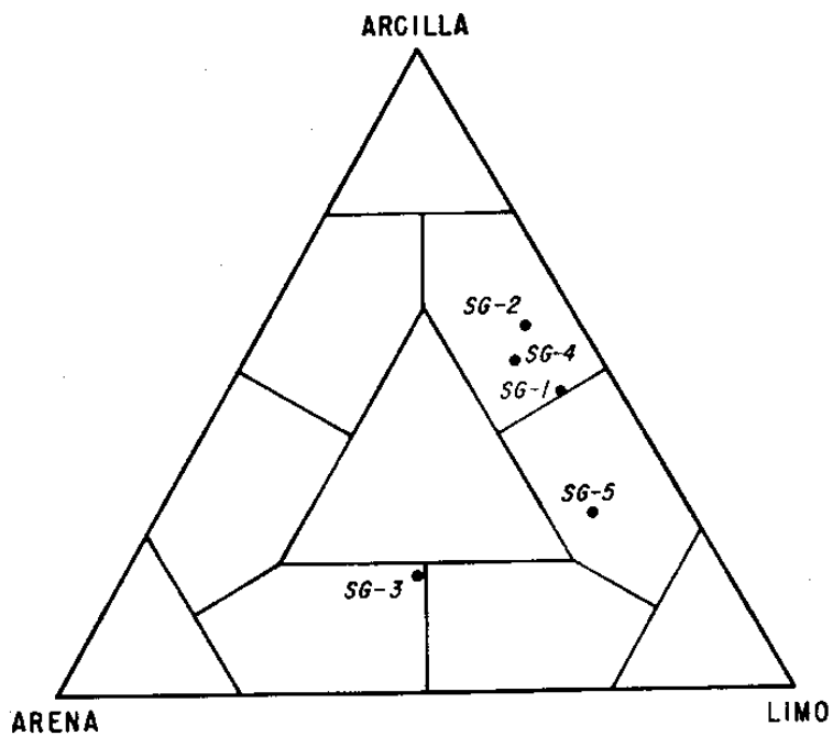
Figura 2.- Distribución del porcentaje de sedimentos según el método propuesto por Shepard (1954).
