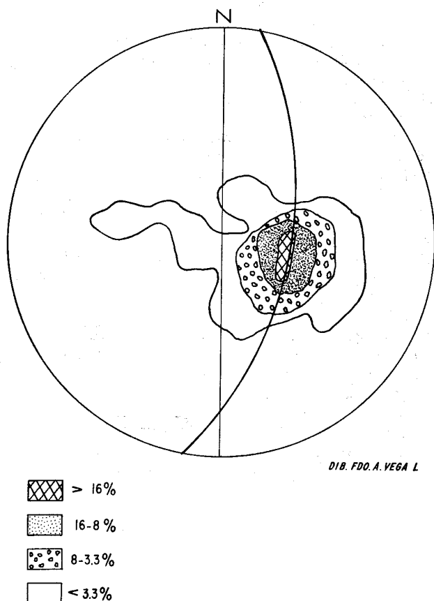
Figura 4.- Diagrama de contornos de polos de 60 mediciones de foliación. La actitud promedio de la estructura general es N10°E-34°W.
