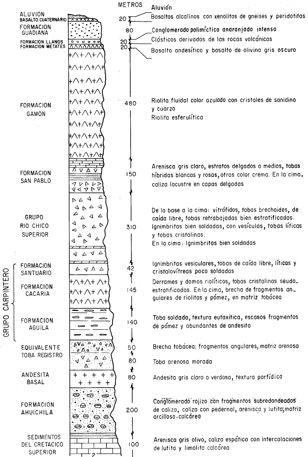
Figura 3.- Columna estratigráfica generalizada del área de las Sierras de Cacaria, San Lucas, La Silla y Gamón.
