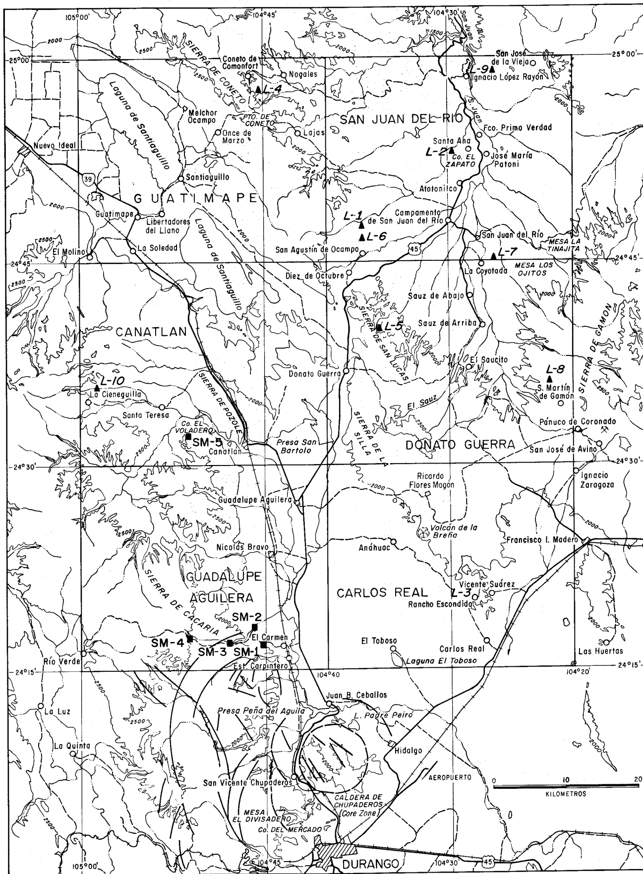
Figura 1.- Mapa de localización del área estudiada, de las secciones medidas (SM-1) y de algunas localidades mencionadas en el texto (L-1).
