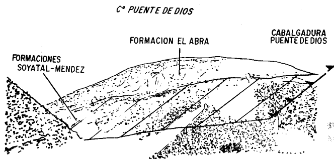
Figura 9.- Panorama en el corte del río Jalpan, visto desde su ribera sudoriental. Las rocas alóctonas son de la Formación El Abra, de la plataforma de Valles-San Luis Potosí.
