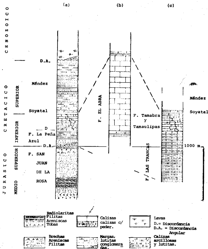
Figura 2.- Columna esquemática de la litoestratigrafía de las rocas mesozoicas. (a) Región al oeste de Peñamiller, (b) región de la plataforma de Valles-San Luis Potosí y banco El Doctor, y (c) cuenca de Zimapán.
