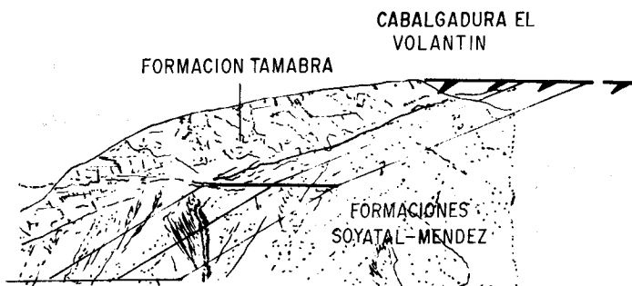
Figura 8.- Cabalgadura El Volantín, en el norte del río Extoraz, vista desde la ribera sur. Las rocas del alóctono son masivas, pero hacia la izquierda de la figura, hay estratos del cantil calcáreo que se truncan contra el Cretácico Superior.
