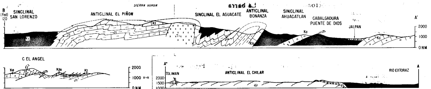
Figura 3.- Sección estructural a través de la Sierra del Pinal. Explicación en el texto.
