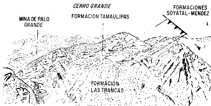
Figura 7.- Panorama del Cerro Grande, visto desde la ribera meridional del río Extoraz; se observa el ángulo aproximadamente recto entre el flanco nororiental y el techo del anticlinal El Piñón.
