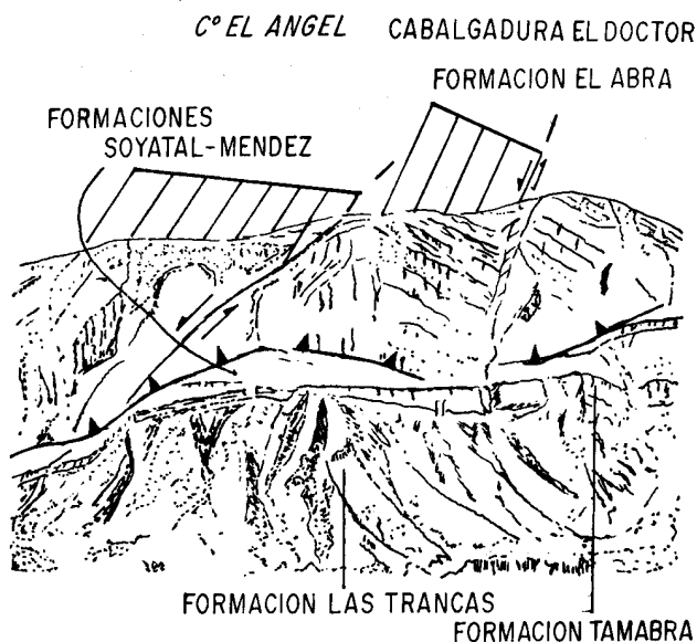
Figura 6.- Panorama del Cerro del Ángel, visto desde el sudeste. La cabalgadura yuxtapone a las facies de borde de plataforma contra estratos de la Formación Tamabra o la Formación Soyatal-Méndez. Se aprecia las fallas de ángulo alto en el alóctono.
