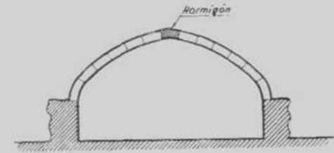
CORTE DE LA HABITACION SUBTERRANEA DE LA TORRE
