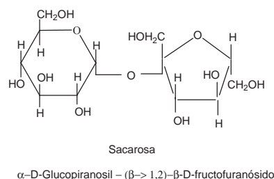
Esquema 4: Estructura del azúcar.
