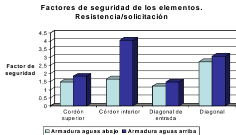
Figura 10. Factores de seguridad de los elementos de las armaduras del puente
