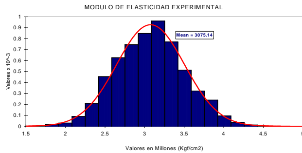
Figura 13. Ajuste de datos simulados de esfuerzo de fluencia
