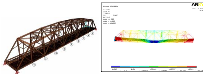
Figura 6. Modelo en SAP-2000 y ANSYS del puente Puerto Salgar
