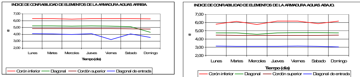
Figura 16. Índices de confiabilidad de los elementos armadura aguas arriba (a) y aguas abajo (b)
