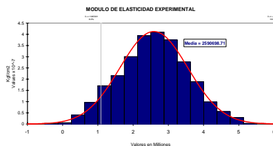
Figura 12. Ajuste de datos simulados de módulo de elasticidad
