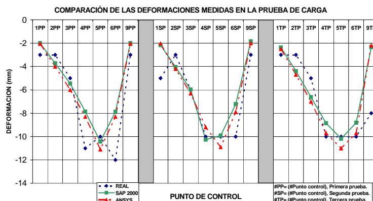
Figura 7. Comparación entre deformación vertical de campo y analítica
