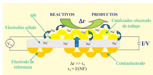
Figura 1. Representaci n esquem tica del efecto NEMCA empleando \text{Na-}\beta\text{-Al}_2\text{O}_3 como s lido conductor.
