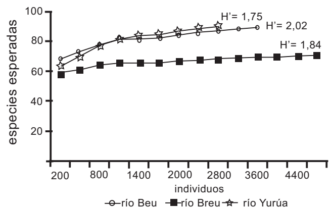
Figura 2. Curva de Rarefacción de especies por Subcuencas en la cuenca del Alto Yurúa.
