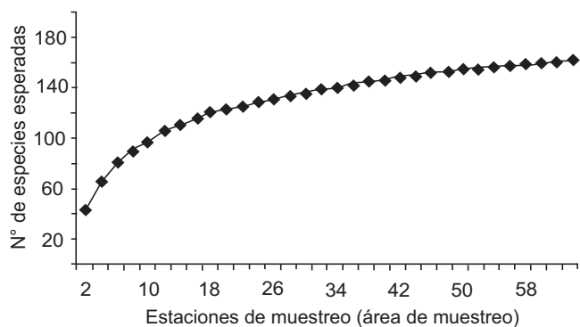
Figura 3. Curva de acumulación de especies según estación de muestreo en la cuenca del Alto Yurúa.
