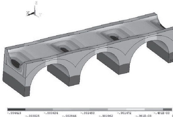
Figura 15. Desplazamientos en el eje Z en la obra de albañilería del puente La Libertad.
