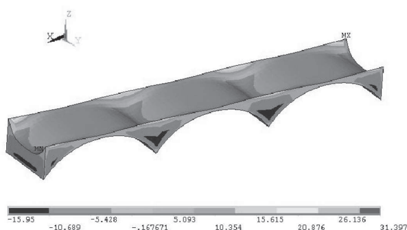
Figura 10. Esfuerzos en el eje Y del material de relleno del puente La Libertad.
