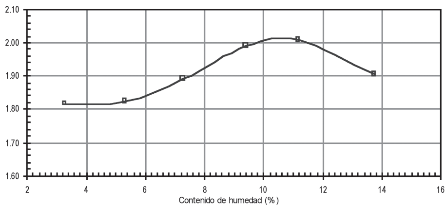
Figura 1. Peso unitario seco en función del contenido de humedad. Resultados típicos obtenidos en un ensayo de compactación proctor.
