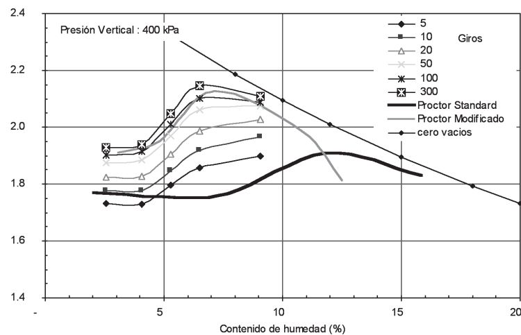
Figura 13. Presión de vertical de 400 kPa
