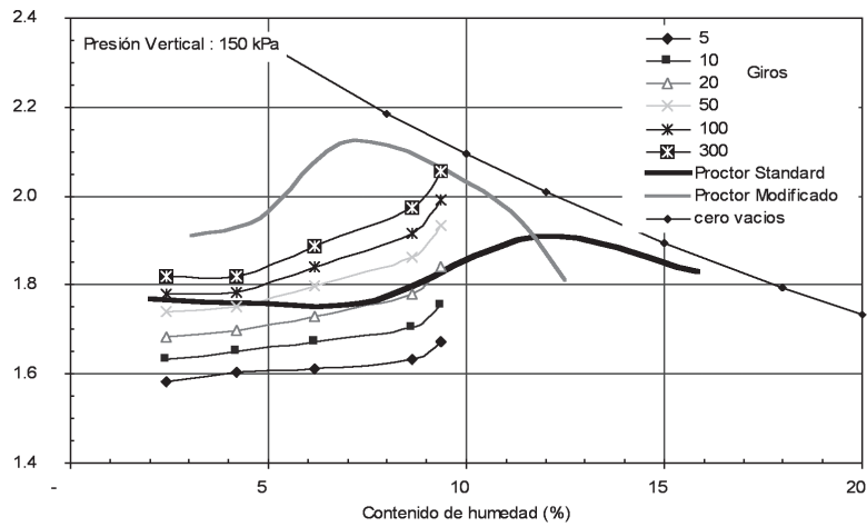
Figura 9. Presión de vertical de 150 kPa
