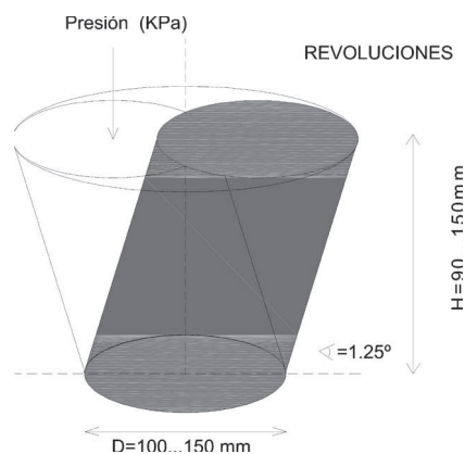
Figura 3. Acciones ejercidas por el equipo de compactación giratoria
