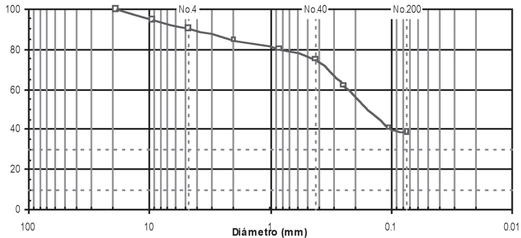
Figura 4. Granulometría del material de granular
