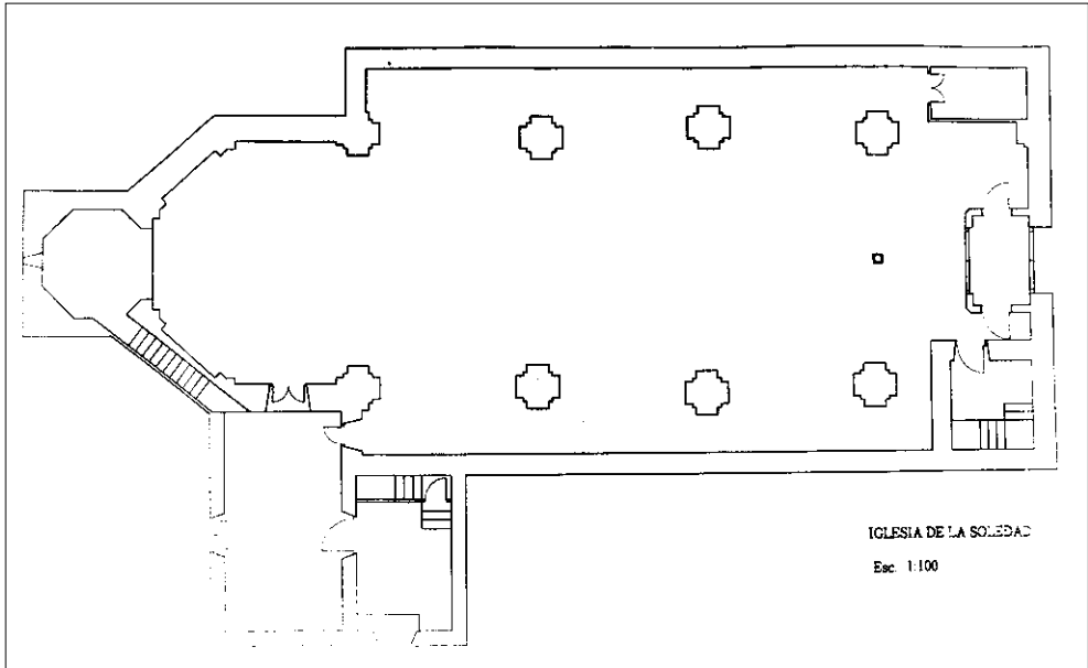
Figura 1. Planta.
