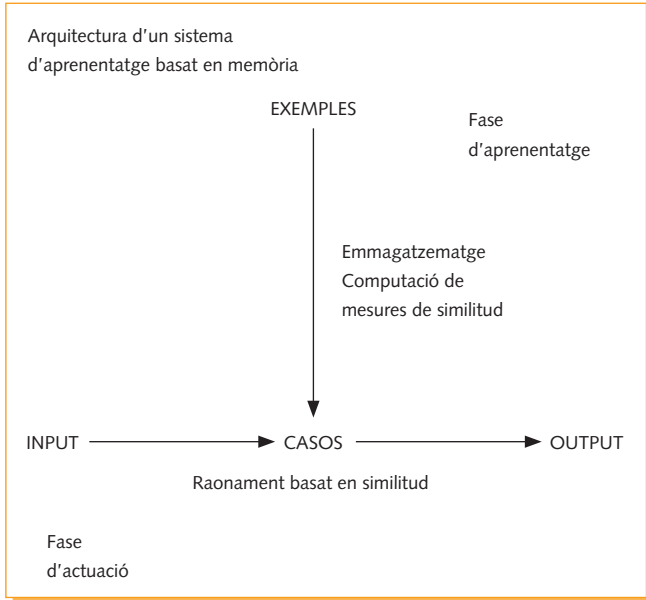
Figura 1. Arquitectura general d'un sistema de MBL (Daelemans et al. , 2007, pàg. 19)
