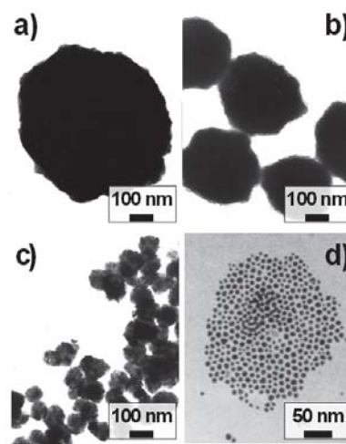
Fig. 6. Imágenes de microscopía electrónica de transmisión (MET) de partículas de \text{Co}_{80}\text{Ni}_{20} preparadas por el método de los polioles que induce a una nucleación heterogénea con núcleos de Ag o Pt: a) partículas de \sim 500 nm ( [\text{Ag}]/[\text{Co}+\text{Ni}] = 1.0 \cdot 10^{-5} ), b) partículas de 320 \pm 30 nm ( [\text{Ag}]/[\text{Co}+\text{Ni}] = 2.5 \cdot 10^{-5} ), c) partículas de 90 \pm 8 nm ( [\text{Pt}]/[\text{Co}+\text{Ni}] = 2.0 \cdot 10^{-5} ), y d) partículas de 5.9 \pm 0.8 nm ( [\text{Pt}]/[\text{Co}+\text{Ni}] = 0.025 ) sintetizadas en presencia de agentes estabilizadores estéricos (ácido oleico).
