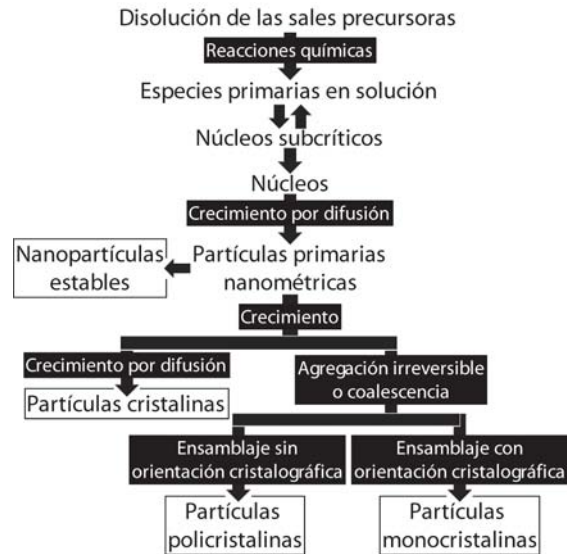
Fig. 1. Etapas de la formación de partículas por precipitación química en soluciones homogéneas.
