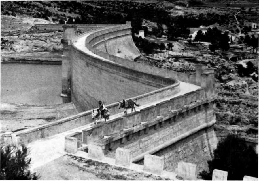
FIG. 1 Presa del embalse de Puentes.
