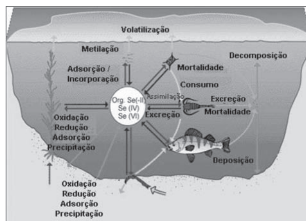
Figura 1. Ciclo biológico do selênio no ambiente aquático (adaptado de Bowie et al. 1998).
