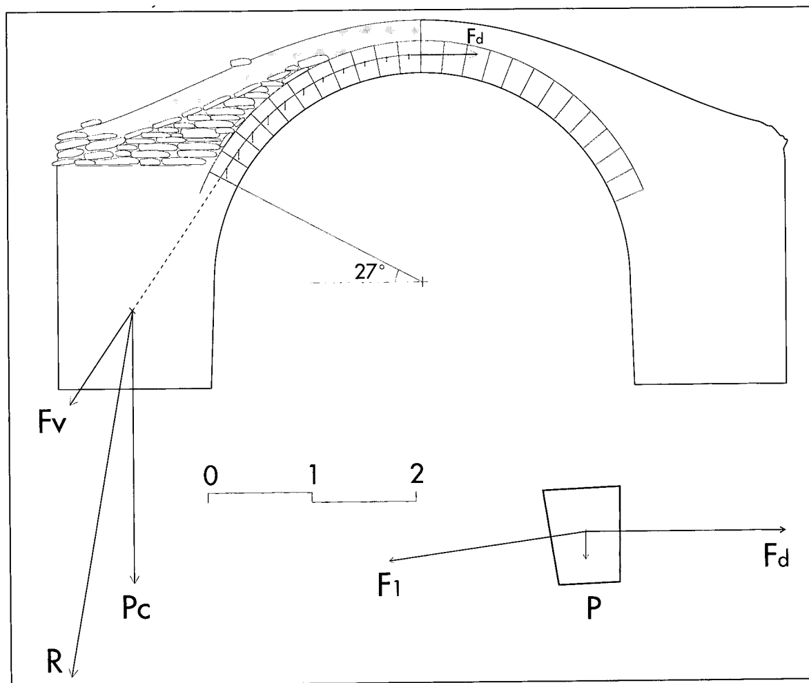
Forces que genera una volta.
