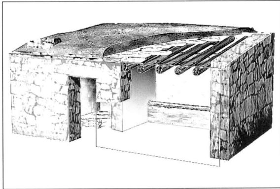
Cabana amb sostre de llosetes. Secció.
