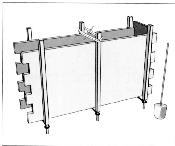
Tapiera amb un captauló.
