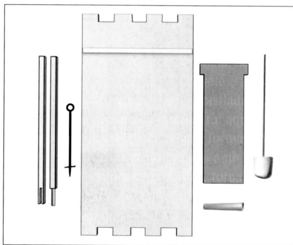
Components de la tapiera.
