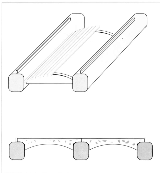
Revoltons de guix.
