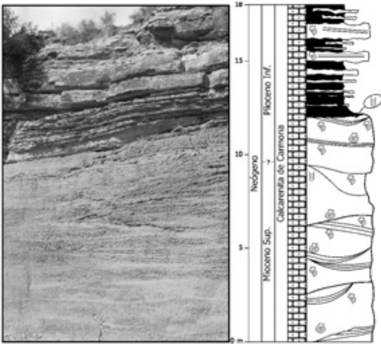
◀ Figura 4. Frente de explotación de la Calcarenita de Carmona y columna estratigráfica correspondiente. Los estratos inferiores pertenecen a los bancos canterables, mientras que los superiores no se explotaban.
