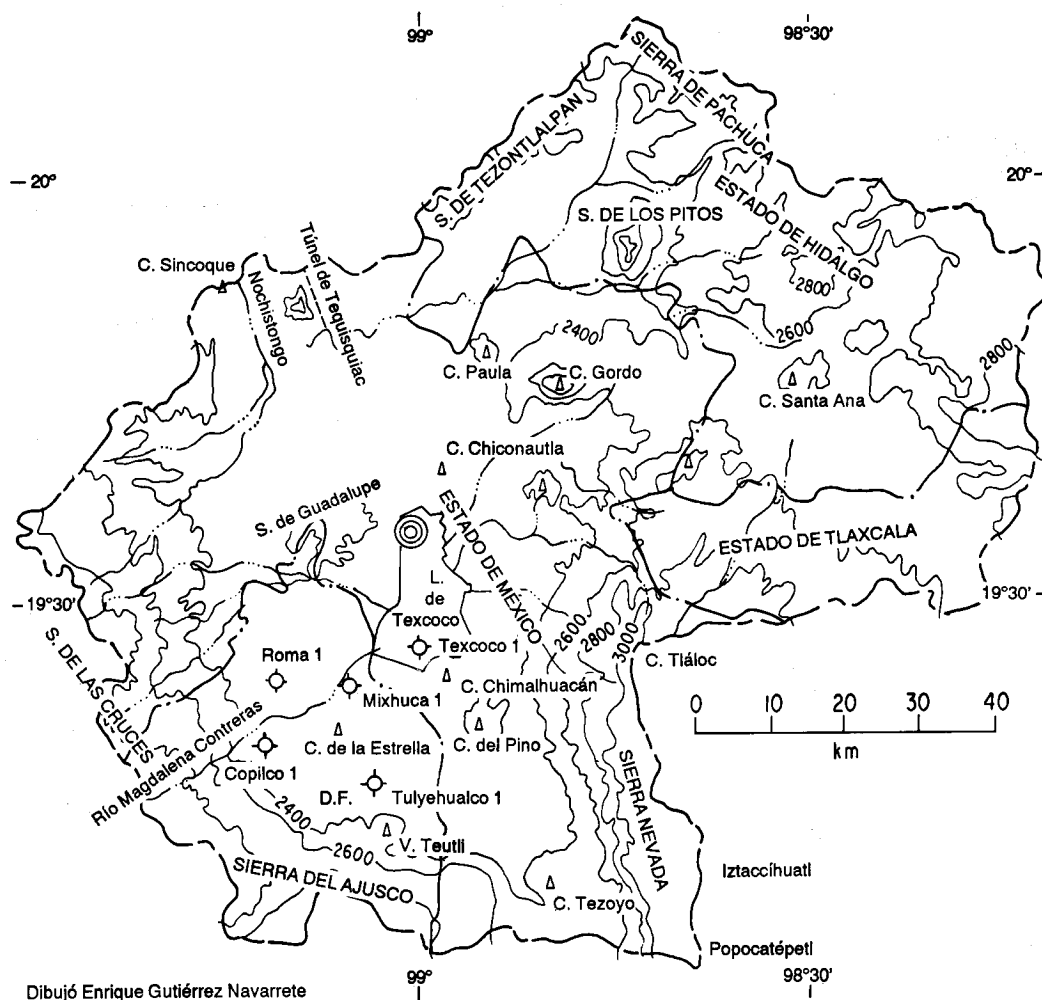
Figura 1.- Mapa fisiográfico del área de estudio en el que se indica los límites de la cuenca de México.
