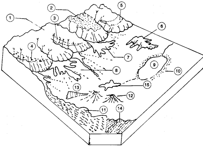
Figura 2.- Bloque diagramático hipotético que muestra los tipos litológicos principales y sus relaciones fisiográficas desde una vista hacia el noroeste. 1, sierras y lomas accidentales; 2, toba pumítica y lapilli; 3, derrames de lava principalmente andesíticos; 4, brecha y aglomerado volcánico; 5, lahar y derrames de ceniza; 6, remanentes de derrames de lava miocénicos; 7, flujos de lodo; 8, abanicos aluviales coalescentes; 9, depósitos lacustres; 10, depósitos de playa; 11, derrames de lava basálticos; 12, conos piroclásticos; 13, derrames de lava basáltica con estructura cordada y túmulos; 14, lavas dacíticas y material piroclástico y clástico; 15, depósitos palustres: turba-diatomita.
