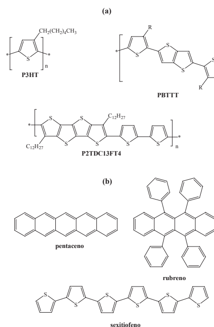
Figura 5. Polímeros conjugados (a) y moléculas conjugadas pequeñas (b) utilizados como semiconductores en OFETs.
