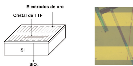
Figura 7. Izquierda: Configuración utilizada para el dispositivo. Derecha: Imagen obtenida por microscopio óptico de un cristal de DT-TTF sobre electrodos de oro. Reproducido con el permiso de la referencia 20a. Copyright 2004 American Chemical Society.
