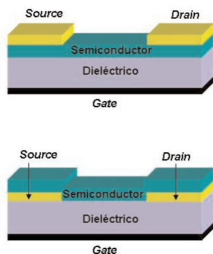
Figura 2. Configuraciones de un OFET: contacto superior (arriba) y contacto inferior (abajo).
