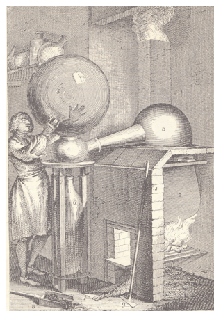
Figura 4. Alrededor de 1740 el curandero inglés Joshua Ward (1685–1761) mejoró notablemente la fabricación de ácido sulfúrico reemplazando la campana por grandes globos de vidrio, los cuales reducían enormemente las pérdidas de gases de \text{SO}_2 y \text{SO}_3 . No mucho después los frágiles recipientes de cristal fueron reemplazados por cámaras de plomo. Fuente: C. Singer, The Earliest Chemical Industry , The Folio Society, London, 1948, p. 274.
