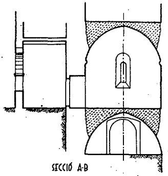
SECCIÓ A-B
