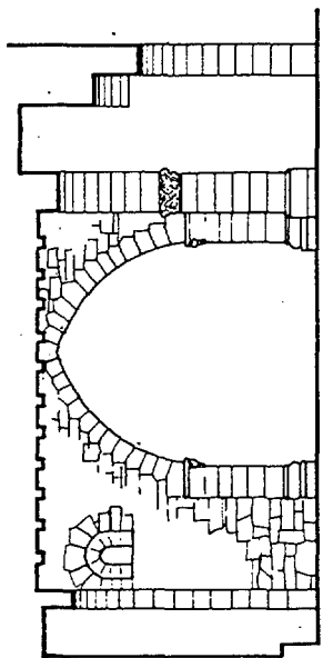
SECCIÓ A-B
