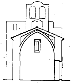
SECCIÓ A-B
