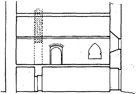
SECCIÓ C-D
