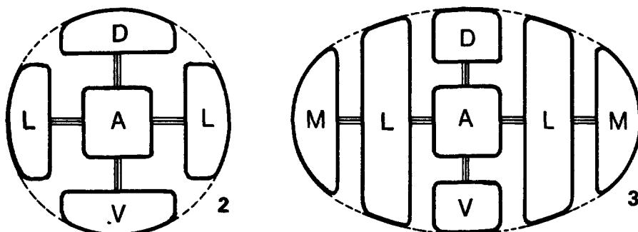
Fig. 2.— Cottoniella filamentosa var. fusiformis . Corte transversal, sección cilíndrica. A: célula axial. L: célula lateral. D: célula dorsal. V: célula ventral.
