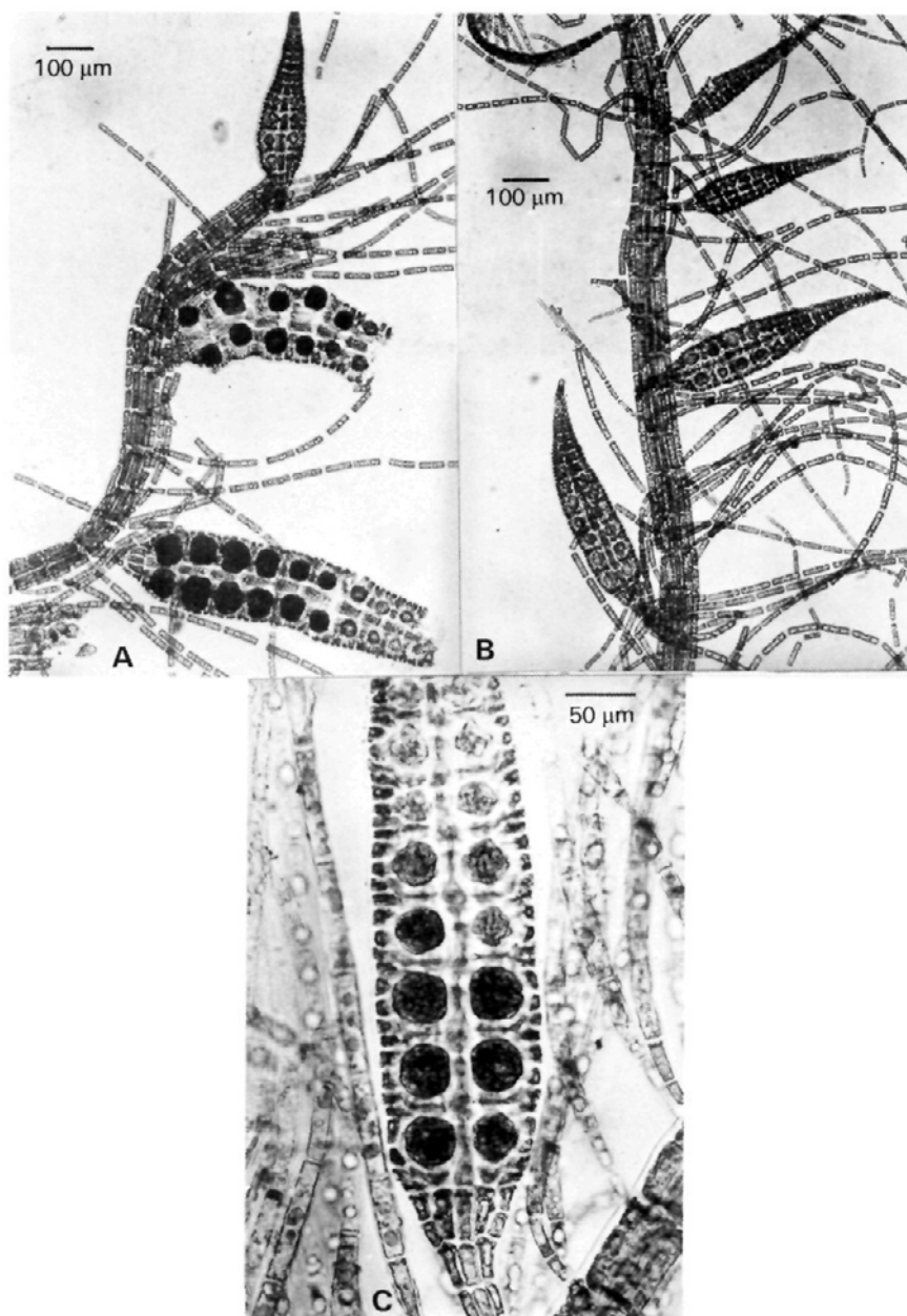
Fig. 6.— Cottoniella filamentosa var. fusiformis . Tetrasporófito. A: Aspecto parcial. B: Estiquidios. C: Detalle de estiquidio con tetrasporocistes.
