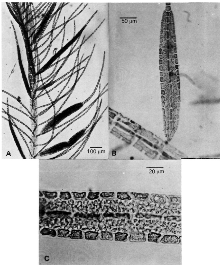
Fig. 7.— Cottoniella filamentosa var. fusiformis . Gametófito masculino. A: Hábito. B: Espermatocistóforo. C: Detalle del espermatocistóforo y células madres de los espermacios.
