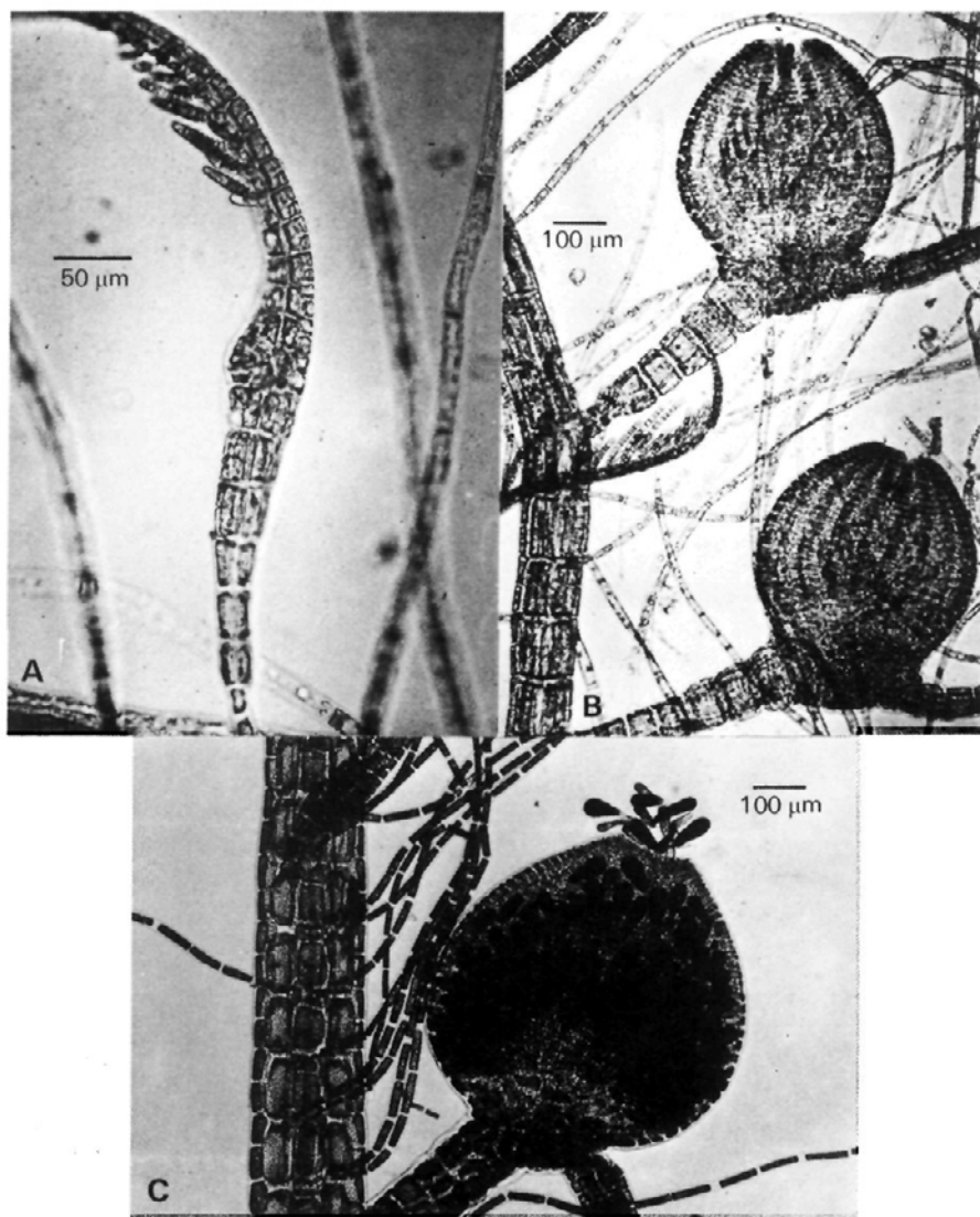
Fig. 8.— Cottoniella filamentosa var. justiformis . Gametófito femenino. A: Primeros estadios del carposporófito. B: Cistocarpos inmaduros. C: Cistocarpos maduros y carposporocistes.
