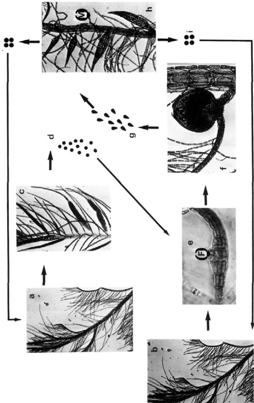
Fig. 9.—Probable ciclo básico de Cottoniella filamentosa var. fusiformis , a: gametofito masculino, b: gametofito femenino, c: rama con espermatocistóforos, d: espermios, e: fase de iniciación del gonimoblasto, f: cistocarpo maduro, g: carposporas, h: tetrasporófito con estiquidos, i: tetrasporas, F: fusión, M: meiosis.
