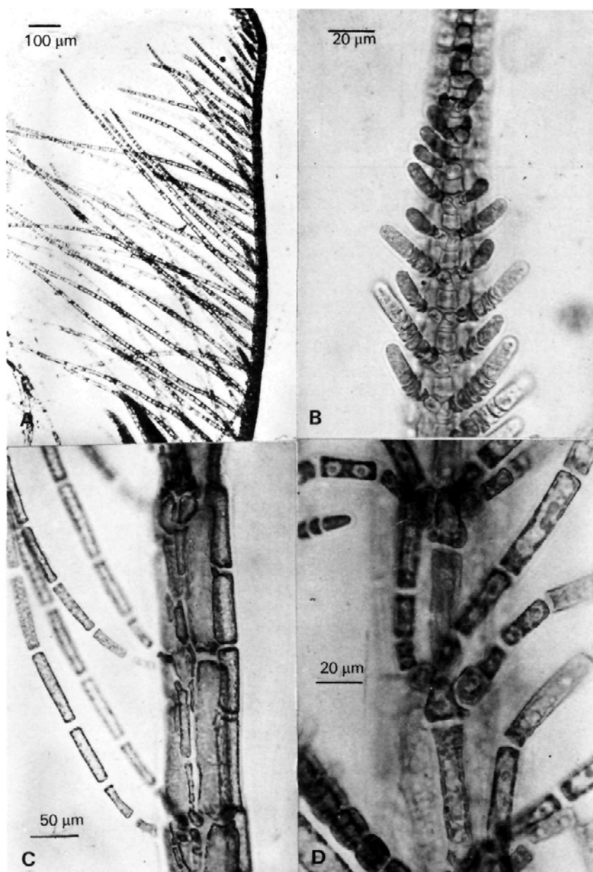
Fig. 5.— Cottoniella filamentosa var. fusiformis . A: Ramas monosifonadas, visión lateral. B: Rama polisifonada con salida de ramas monosifonadas, visión ventral. C: Salida de dos ramas monosifonadas por segmento, visión lateral. D: Salida de tres ramas monosifonadas por segmento, visión ventral.
