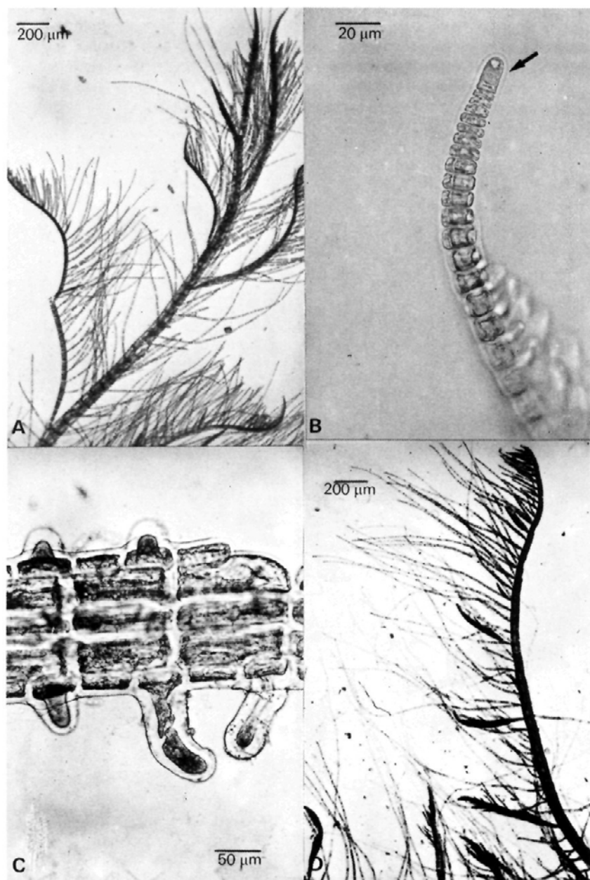
Fig. 4.— Cottoniella filamentosa var. fusiformis . A: Hábito. B: Célula apical de una rama polisifonada. C: Filamentos rizoidales. D: Ramas poli y monosifonadas.
