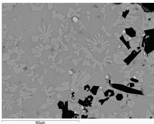
Figura 4. Detalle de la estructura cristalina de la escoria adherida a la superficie interna de un crisol, bajo el microscopio electrónico de barrido. En este caso, los residuos se corresponden con el procesado de una tetraedrita argentífera ( \text{Cu}_{12}\text{Sb}_4\text{S}_{13} ).
