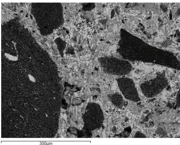
Figura 7. Microestructura de una copela usada bajo el microscopio electrónico de barrido. Además de los granos de cenizas (gris oscuro), que muestran la característica estructura esponjosa del hueso, puede apreciarse la gran cantidad de litargirio (PbO, gris claro) absorbida por el cuerpo de la copela.
