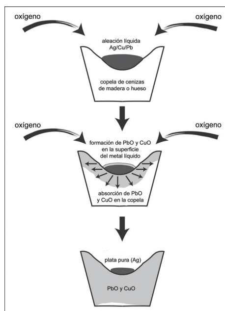
Figura 6. Esquema explicativo del proceso de copelación. En este ejemplo, durante el proceso de refinación por oxidación, la plata se separa de cobre y plomo (Cortesía de Nicolas Thomas).
