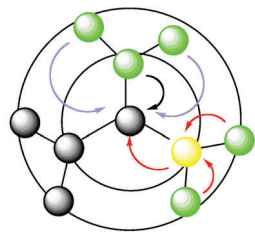
Figura 5. Mecanismo de transferencia de energía.
