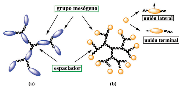
Figura 7. a) Estructura de un dendrímico con unidades mesógenas en las ramificaciones. b) Estructura de un dendrímico con unidades mesógenas en la periferia con los elementos que los constituyen: matriz dendrímica, espaciador y unidades mesógenas (unidas lateral o terminalmente al dendrímico).
