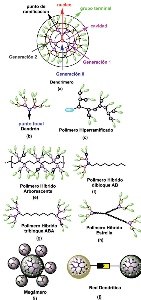
Figura 1. Representaci n esquem tica de diferentes tipos de pol meros dendr ticos y macromol culas h bridas dendr ticas-lineales.
