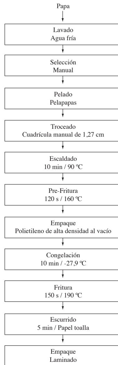
Fig. 1. Proceso de elaboración de papas prefritas congeladas a escala piloto.
