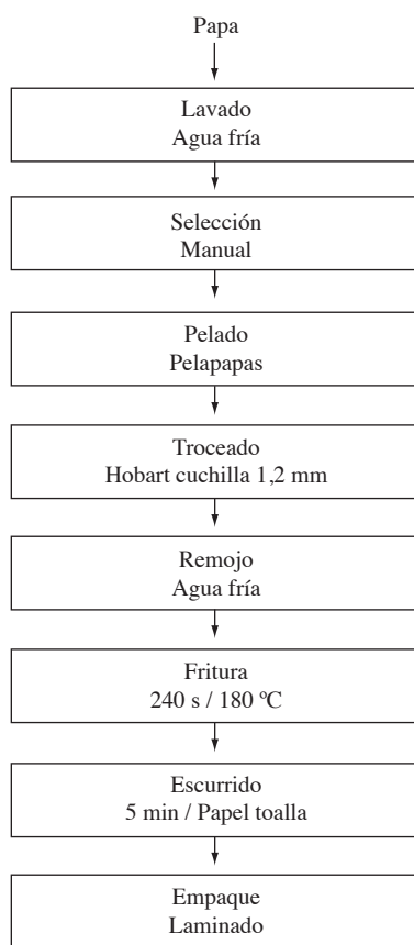
Fig. 2. Proceso de elaboración de papas tostadas a escala piloto, de acuerdo con Añon (1984).
