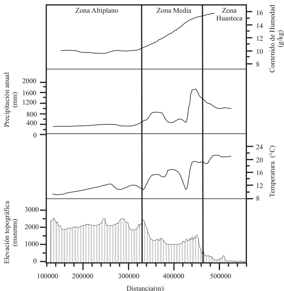
Figura 4. Sección transversal Oeste-Este (latitud norte: 22.05°) de perfiles de (a) humedad relativa media anual, (b) precipitación acumulada media anual, (c) temperatura media anual y (d) elevación de terreno. La sección muestra un corte del Altiplano hacia la zona Huasteca, en las zonas bajas costeras, en un gradiente topográfico pronunciado.
