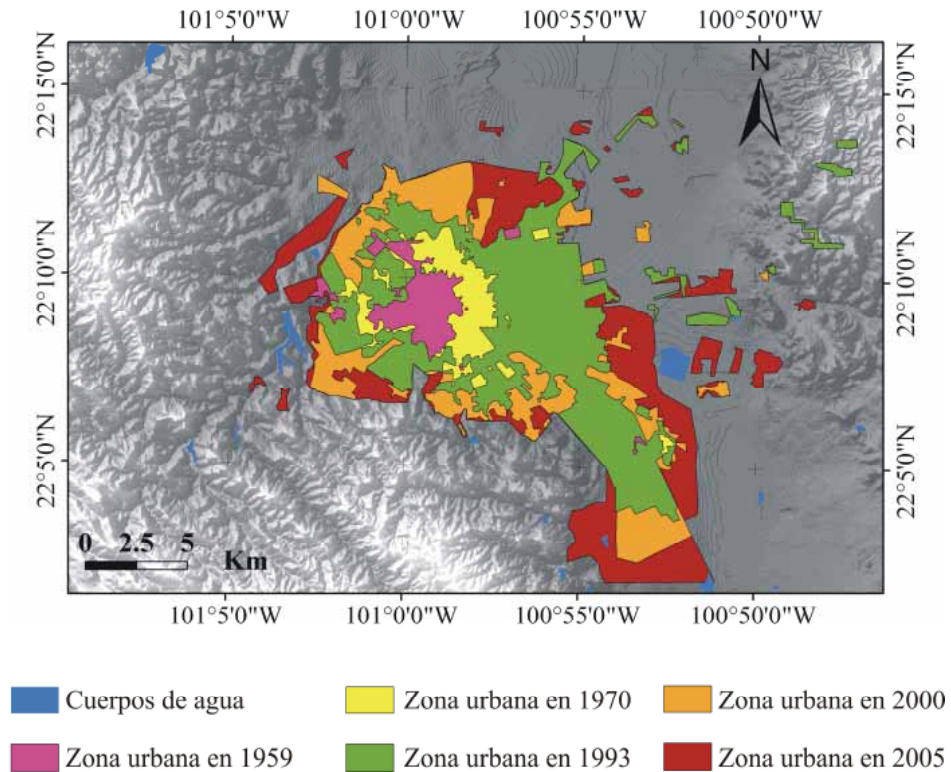
Figura 9. Crecimiento urbano registrado de 1959 a 2005 para la ciudad de San Luis Potosí y área conurbana. La imagen de base es un modelo digital de elevación en tonos de gris.
