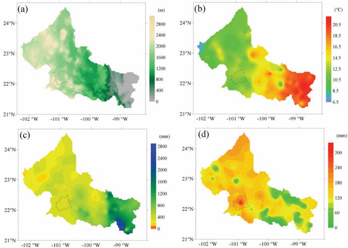
Figura 5. Distribución horizontal de (a) elevación de terreno, (b) temperatura media anual, (c) precipitación media anual y (d) evaporación media anual en el Estado de San Luis Potosí. El contorno interior indica la localización del Valle de San Luis Potosí.
