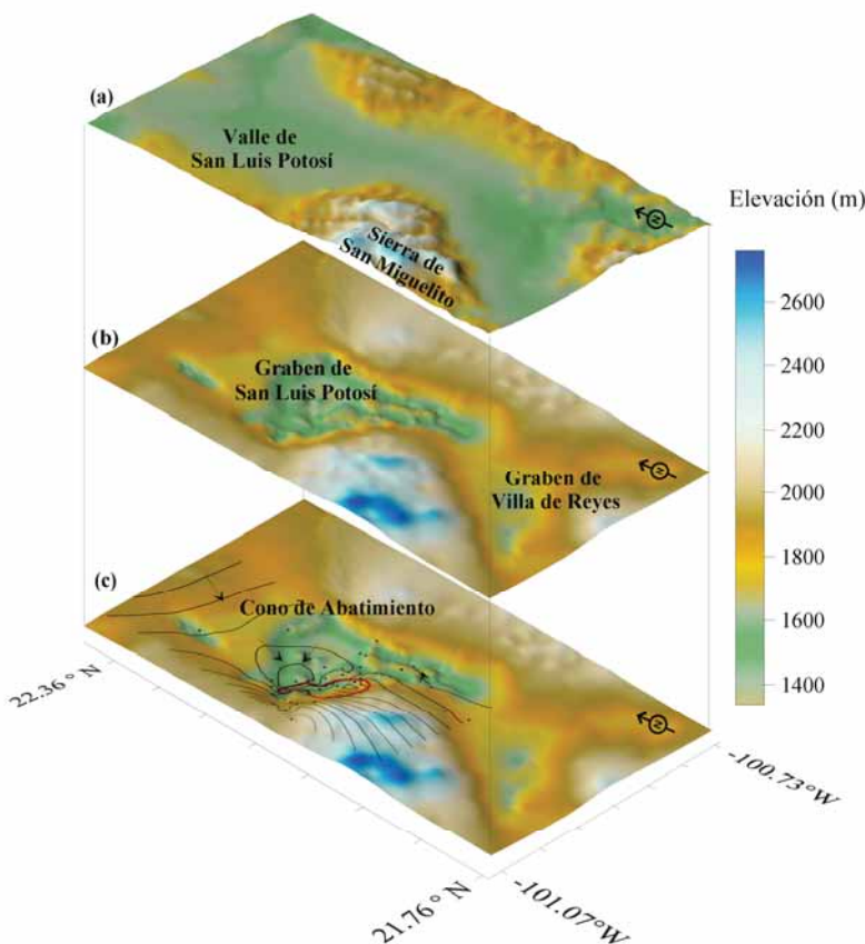
Figura 3. Geometría del subsuelo de la región del Valle de San Luis Potosí y del Valle de Villa de Reyes. a: Elevación topográfica; b: base rocosa del graben de San Luis Potosí y de Villa de Reyes; y c: base rocosa y cono de abatimiento (isopiezas); el contorno rojo indica la zona termal.
