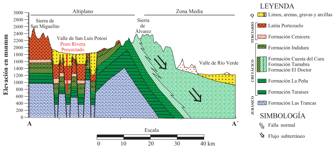
Figura 7. Sección Oeste-Este del Valle de San Luis Potosí (VSLP). La sección corresponde a un corte geológico que va de la Sierra de Álvarez a la Sierra de San Miguelito (la ubicación se muestra en la figura 6). El límite oeste del VSLP es la Sierra de San Miguelito y el límite este es la Sierra de Álvarez. En la figura se muestra la distribución de unidades carbonatadas de baja conductividad hidráulica en el graben del VSLP y rocas con mejores características hidráulicas en la zona media. Se puede observar la presencia de fallas normales formando fosas y pilares dentro del valle. A partir de la estratigrafía de la región, bajo las rocas calcáreas de las formaciones Indidura y Cuesta del Cura, pueden localizarse formaciones como la Peña, Taraises y las Trancas, cuyas característica común es la presencia de material arcilloso y en consecuencia su baja permeabilidad.
