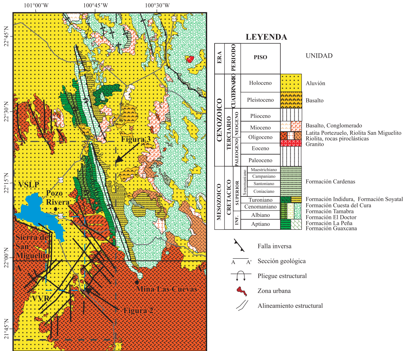
Figura 6. Mapa geol3gico de los valles de San Luis Potos3 y Villa de Reyes (modificado de Labarthe-Hern3ndez et al. , 1982). En la figura se muestran recuadros con l3nea discontinua que corresponden a la localizaci3n de las figuras 2 y 3 y la l3nea continua (A-A') es la secci3n mostrada en la Figura 7.
