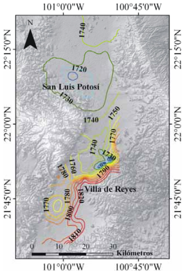
Figura 8. Líneas piezométricas de los valles de San Luis Potosí (VSLP) y de Villa de Reyes. Se observa un mayor abatimiento en la zona del centro del VSLP, donde se localiza la zona urbana de la ciudad de San Luis Potosí. La base de este mapa corresponde al modelo digital de elevación de la zona mostrado en tonos de gris.
