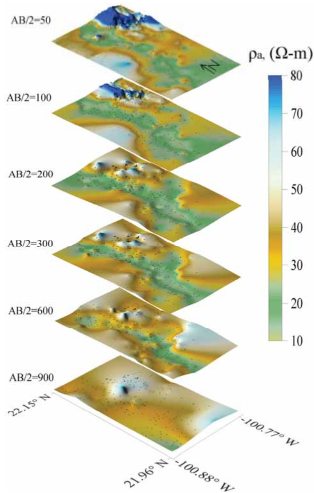
Figura 2. Configuraciones horizontales de resistividad aparente, \rho_a ( \Omega -m), en el VSLP, con espaciamientos de electrodos de corriente (AB/2) de 50, 100, 200, 300, 600 y 900 metros.
