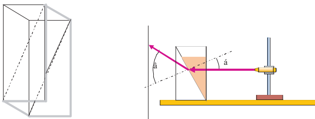
Figura 4. Esquema del refractómetro y de su utilización. Obsérvese que el calibrado debe hacerse en cada utilización, cuidando siempre de reponicionar correctamente la celda.
