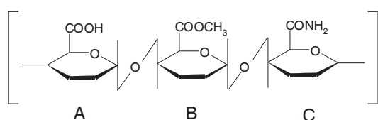
Figura 2. Esquema de una pectina; se observa c mo en el anillo B el grupo carboxilo est  metilado y en el C est  amidado. Por claridad, se omiten los detalles no necesarios, que pueden apreciarse en la Figura 1.
