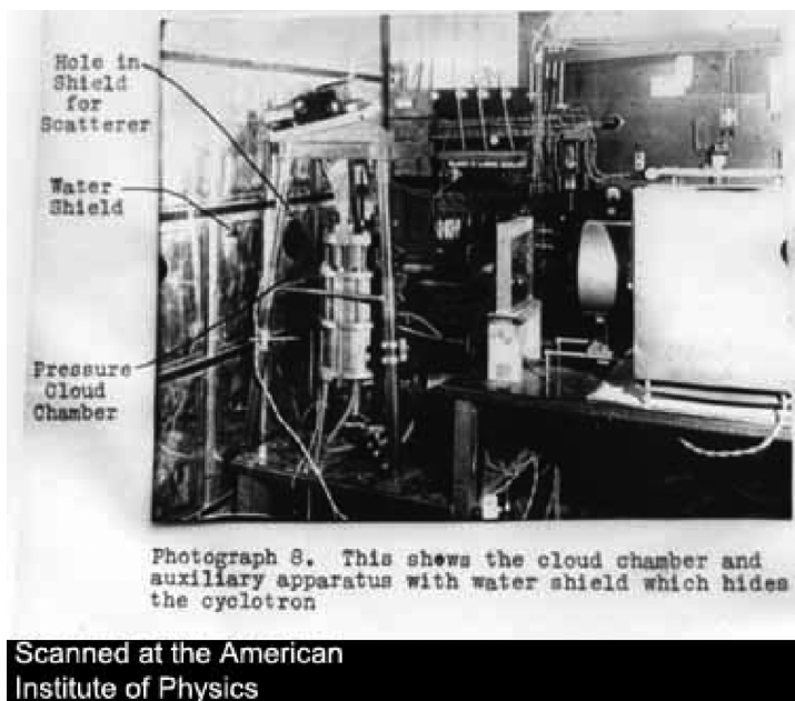
Figura 3. Cámara de niebla conectada a un ciclotrón (AIP Emilio Segre Photo Archive).
