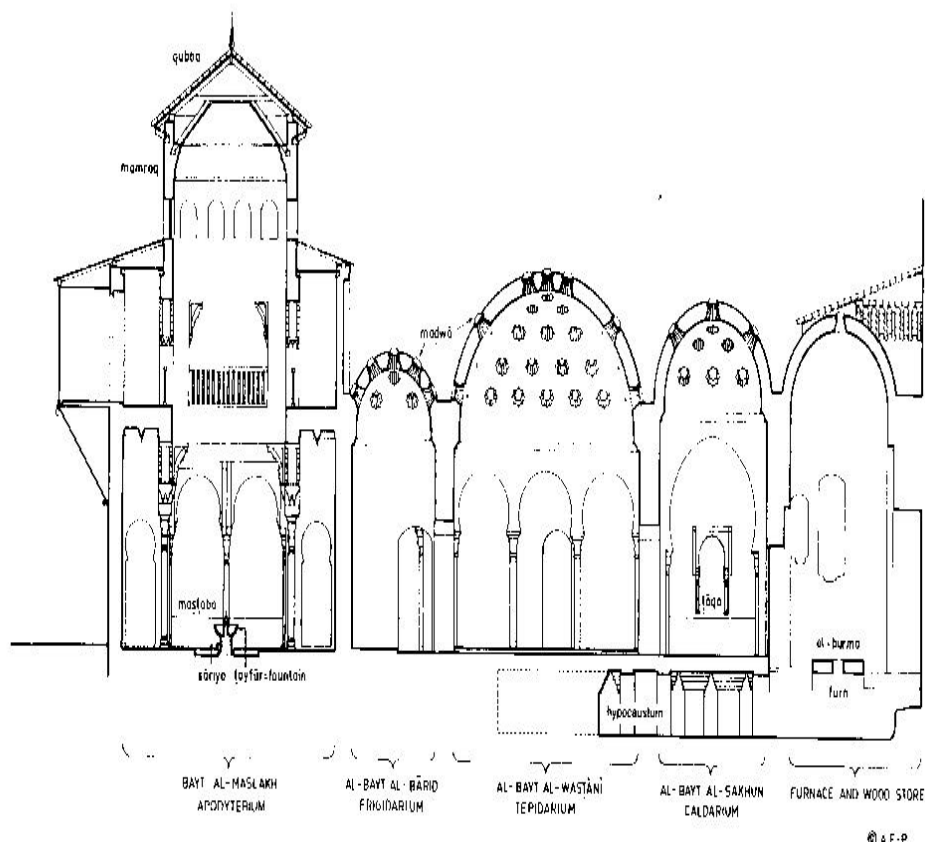
Lámina XXI. Planta y alzado de los baños de Comares. Fernández Puertas, A. The Alhambra .
