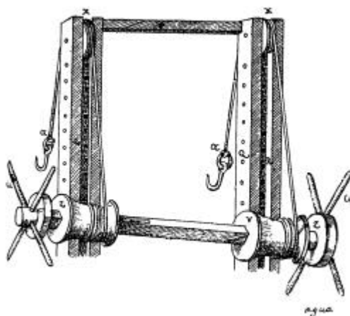
Figura 2. Ingenio utilizado para elevar pesos en El Escorial en el siglo XVI. Fuente: ibídem.
