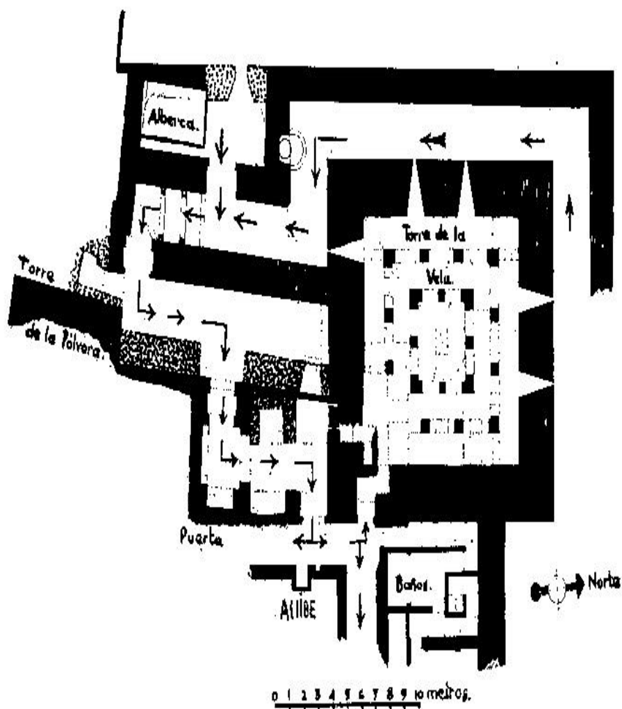
Lámina VI. La torre de la Vela en la Alcazaba. Las flechas indican los accesos desde las caballerizas y del revellín de artillería pasando por dos puertas en recodo hasta llegar a barrio Castrense y los baños. Pavón Maldonado.
