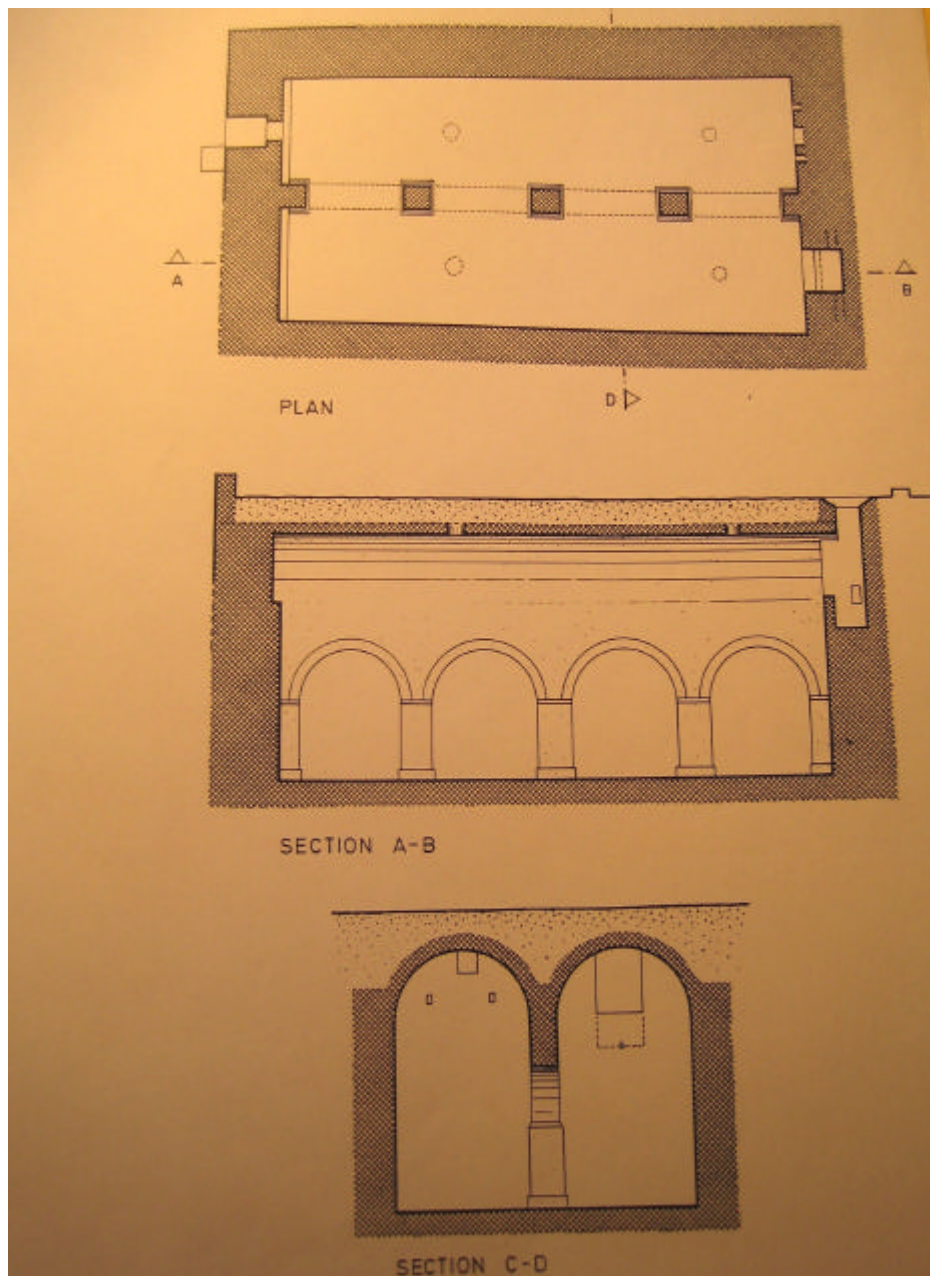
Lámina XII. Planta y alzado del aljibe cristiano del siglo XV y XVI. Fernández Puertas, A. The Alhambra .
