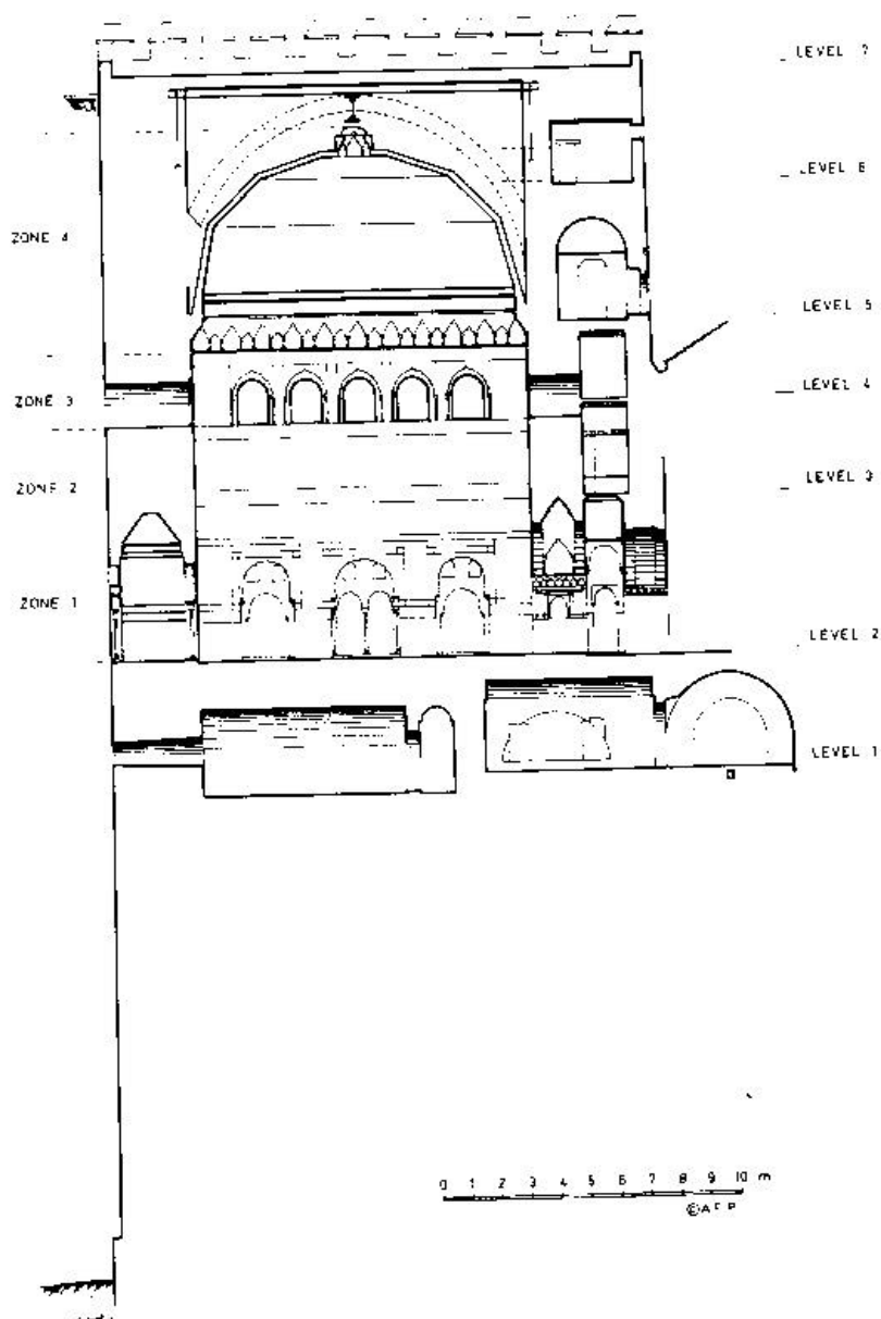
Lámina XXII. Alzado de la torre de Comares según Fernández Puertas.
