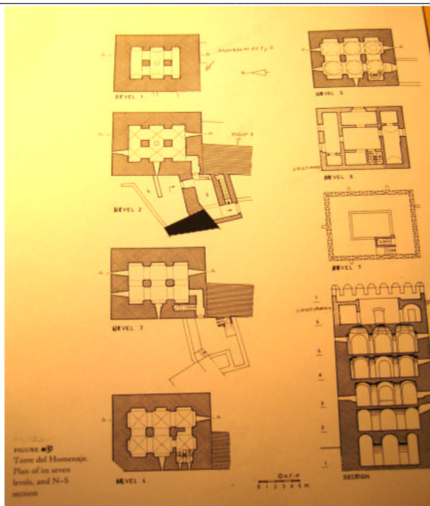
Lámina III. Niveles de la Torre del Homenaje. En el segundo nivel se puede apreciar la puerta en recodo por la que se entra al Barrio Castrense –niveles 2 y 3. Fernández Puertas, A. The Alhambra .
