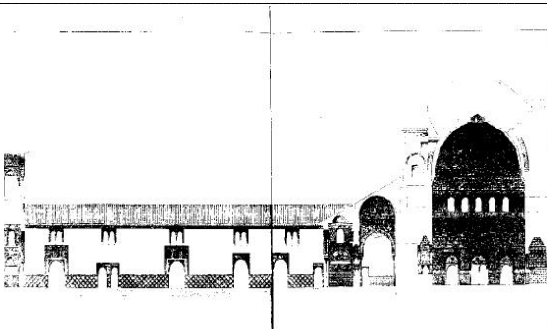
Lámina XIX. Corte transversal de patio de los Arrayanes, el Harem (a la izquierda) y la torre de Comares a la derecha. En ella se aprecia la tipología clásica del palacio nazarí: patio con alberca central, pórtico, nave transversal (Sala de la Barca) y pasillo de separación entre ésta y el Salón del Trono con el oratorio y el acceso a las habitaciones altas. Fernández Puertas, A. The Alhambra .
