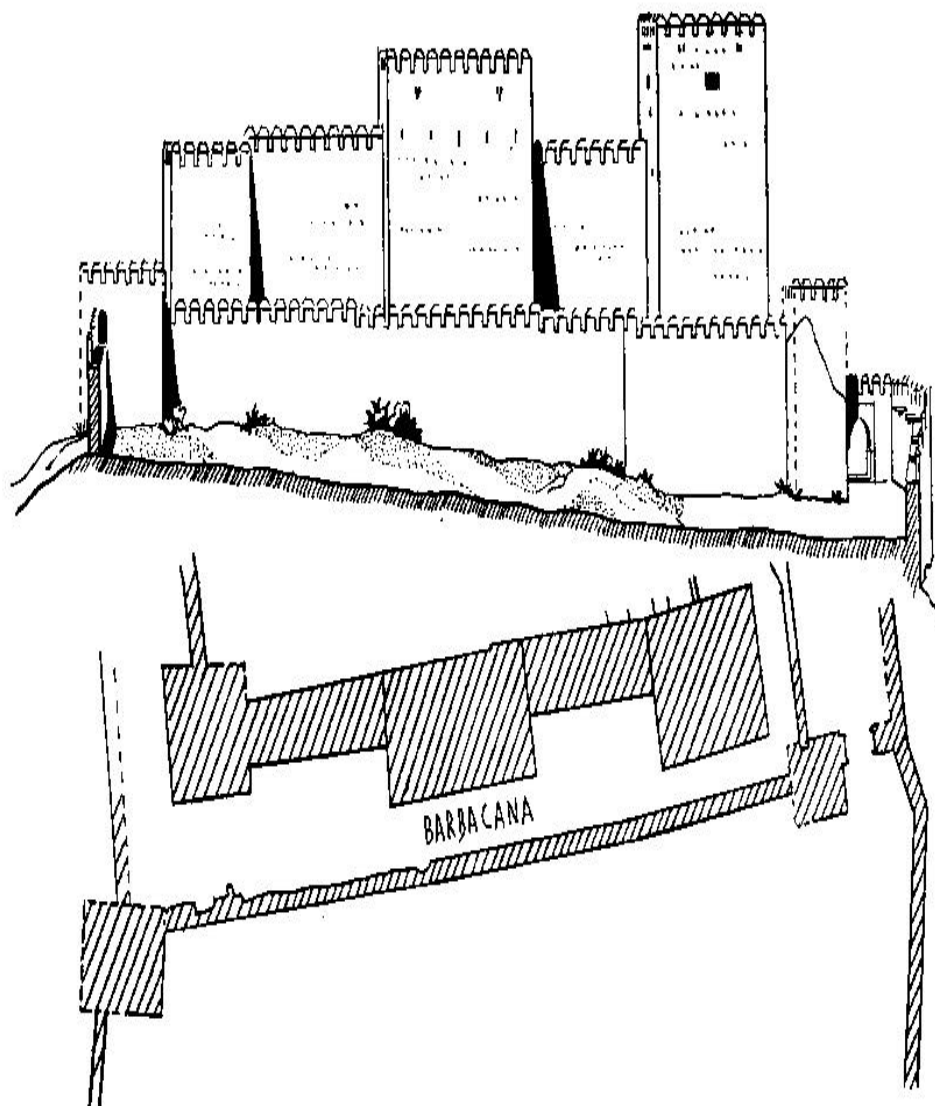
Lámina VIII. Restitución del frente oriental de la Alcazaba. Véanse las dos torres de vigilancia, ya destruidas, que flanquean esta fachada: la puerta de la Tahona (a la derecha), desaparecida al realizar el cubo cristiano, y otra torre (izquierda) delante de la entrada de lo que hoy conocemos como Jardín de los Adarves (cristiano). Pavón Maldonado, Basilio.
