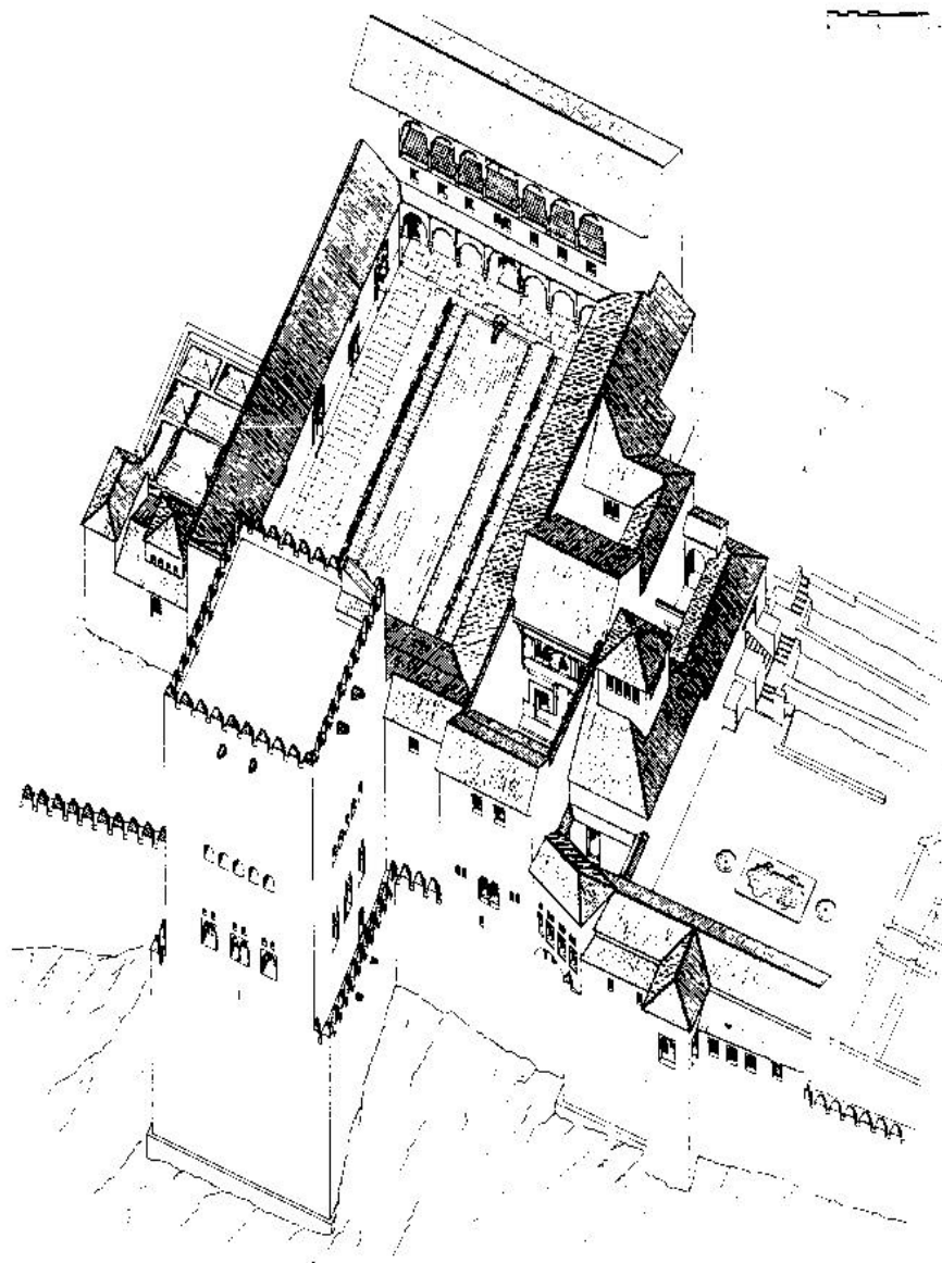
Lámina XVI. Axiometría realizada por Fernández Puertas, A. The Alhambra . Apreciamos La torre de Comares, el Patio de los Arrayanes y la disposición primitiva del Mexuar. Vemos el patio a cielo abierto que daba acceso a otro, el del Salón Dorado al que se entraba desde la Galería de Machuca por una pequeña puerta.
