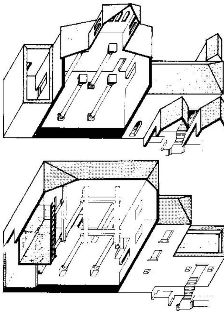
Axonometrías del mexuar en la época nazarí (arriba) y en la cristiana (abajo)
