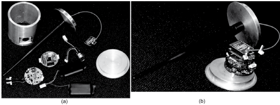
Figura 3. Nodo sensor desarrollado. (a) Partes constitutivas del nodo. (b) Nodo totalmente ensamblado
