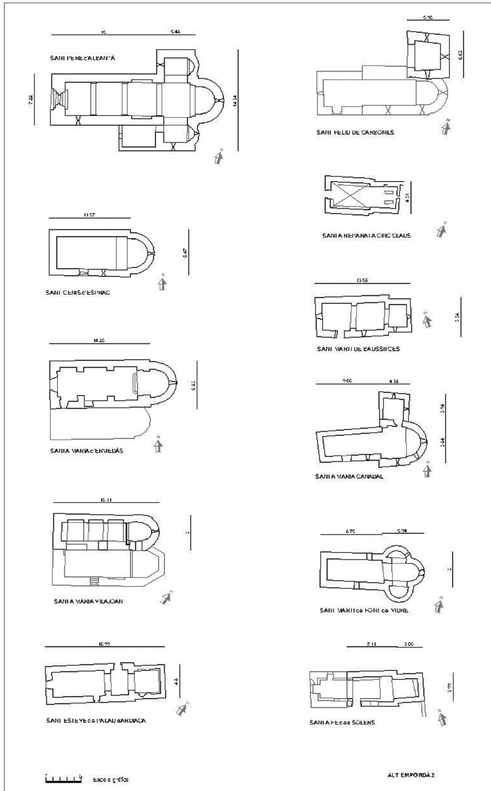
Fig. 4. Planimetrías de trabajo vectorizadas en AutoCad de las iglesias del Alt Empordà (2) (CARE-Hispania, elaboración M. Valls)
