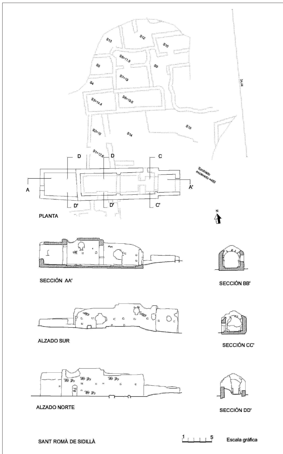
Fig. 5. Planimetrías de trabajo a partir de la documentación existente (Adell, Badía i Homs y Barral) y de la revisión planimétrica de la iglesia de Sant Romà de Sidillà (Foixà, Girona) (CARE-Hispania, elaboración M. Valls)
