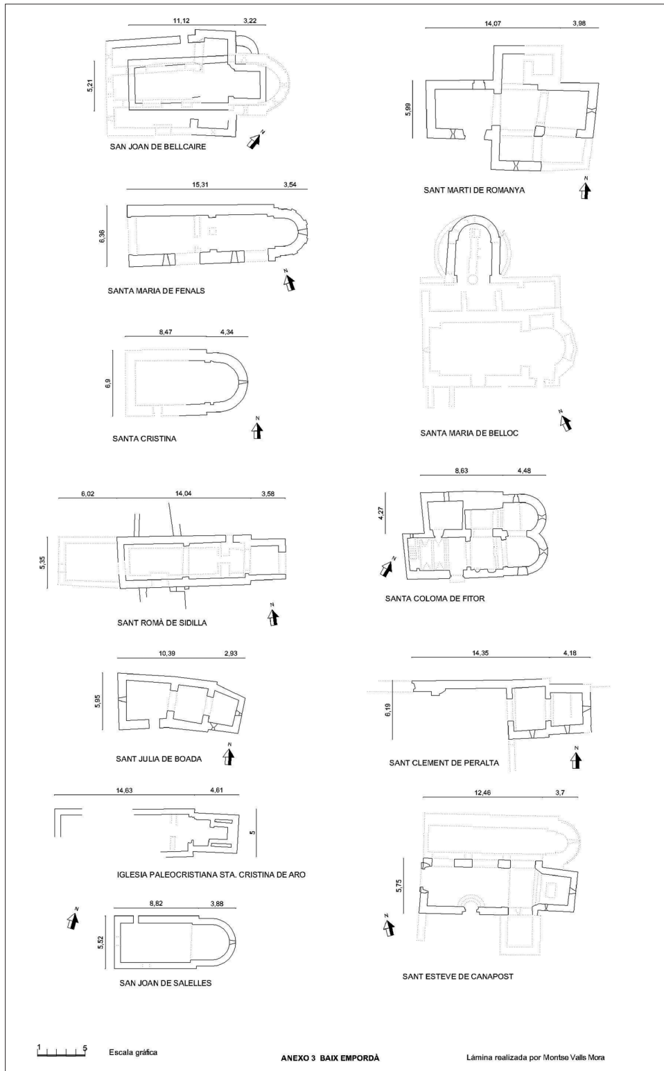
Fig. 2. Planimetrías de trabajo vectorizadas en AutoCad de las iglesias del Baix Empordà (CARE-Hispania, elaboración M. Valls)
