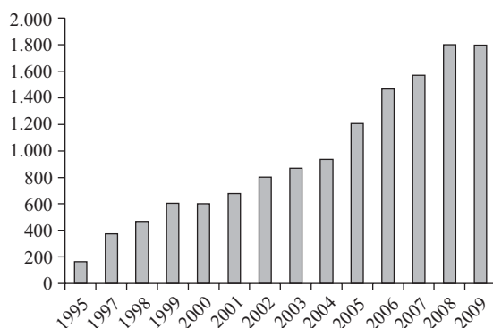
Gráfica 3.- Potencia media anual dos aerogeneradores instalados en Galicia
