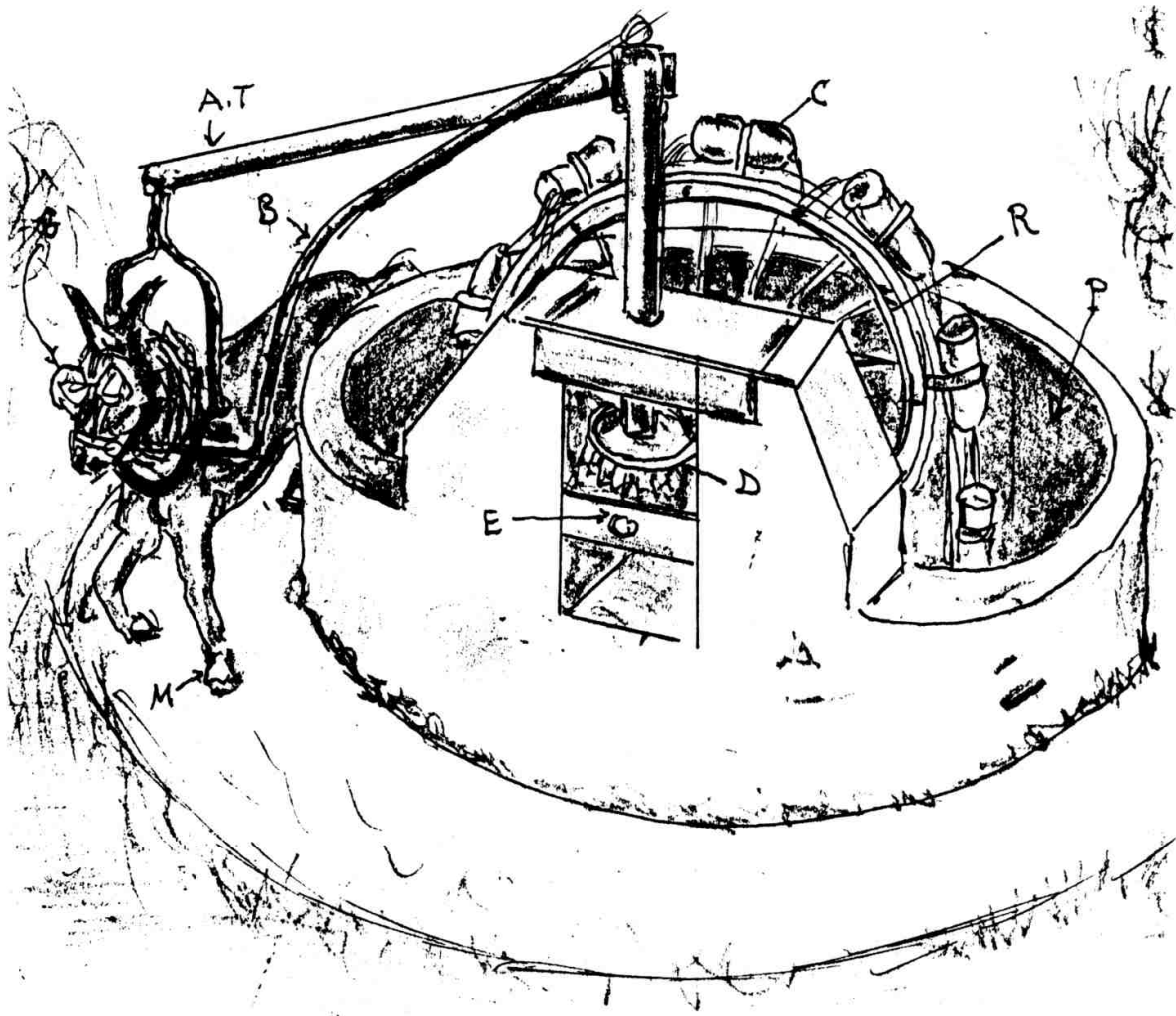
Una sinia de catufols, com la que hi havia a Torredembarra, al darrere de casa.
