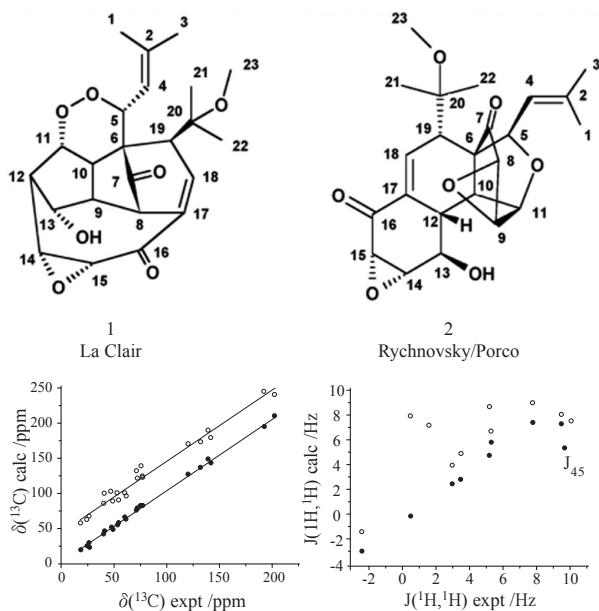
Figura 14. Estructuras propuestas por La Clair y por Rychnovsky/Porco para el hexacyclinol. Abajo, izquierda, \delta 's ( ^{13}\text{C} ) calculadas y observadas para 1 (sin relleno) y 2 (con relleno). La escala vertical está desplazada para 1, por claridad. RMSDs: para (1) 4,1 ppm; para (2) 7,1 ppm. Abajo, derecha, J_{\text{HH}} calculadas y observadas. La señalada con J_{45} puede venir afectada por un equilibrio conformacional.
