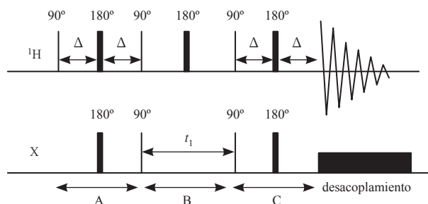
Figura 5. Secuencia de pulsos para el experimento HSQC 17 de correlación de ^1\text{H} con un heteronúcleo.
