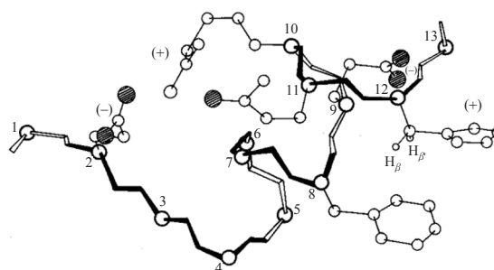
Figura 1. Arriba: asignación de los protones \text{H}_\alpha del fragmento N-terminal de 19 residuos de la enzima Ribonucleasa. Abajo: modelo que satisface todas las observaciones respecto a las variaciones espectrales con el pH y la temperatura. La estructura helicoidal coincide con la que el fragmento adopta en la proteína intacta.
