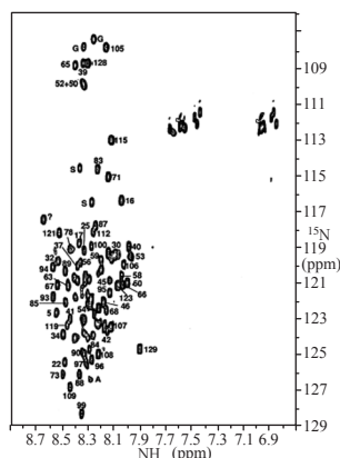
Figura 6. Espectro HSQC ^1\text{H} – ^{15}\text{N} de la proteína Che Y (129 aa) 19 etiquetada uniformemente con ^{15}\text{N} . Arriba: la forma nativa. Abajo: la forma desnaturada en 6M urea. Las escalas de los espectros, horizontal ( ^1\text{H} ), y vertical ( ^{15}\text{N} ) son aproximadamente equivalentes. Obsérvese la gran diferencia en la dispersión de señales en ambas dimensiones.
