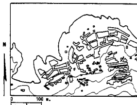
Fig. 8. Adaptación de la trama urbana a la planta de abanico de la isla baja (Villa de Garachico, Tenerife).
