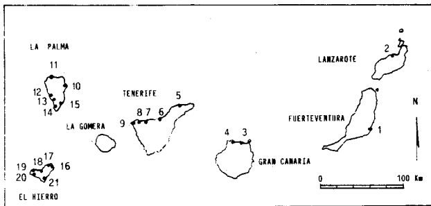
Fig. 1. Localización de las principales islas bajas en Canarias. 1.-Jacomar. 2.-Caletón de las Animas. 3.-Bañaderos. 4.-Galdar. 5.-Punta del Hidaigo. 6.-Puerto de la Cruz. 7.-Garachico. 8.-Daute. 9.-Teno Bajo. 10.-Puntallana. 11.-Juan Adalid. 12.-San Juan. 13.-El Charco-Jedey. 14.-San Antonio-Tenegüfa. 15.-Martín. 16.-Tamaduste. 17.-Las Calcosas. 18.-El Golfo. 19.-Hoya del Verodal. 20.-Orchilla. 21.-La Restinga.
