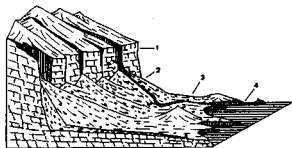
Fig. 2. Unidades topográficas de una isla baja. 1.-Escarpe. 2.-Talud. 3.-Plataforma central. 4.-Frente litoral.
