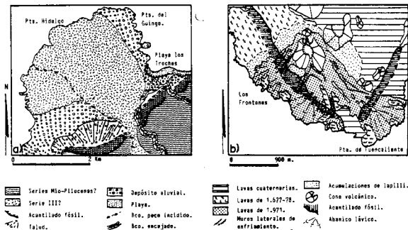
Fig. 5. Diferencias morfológicas entre plataformas costeras antigua y reciente. a) Plataforma antigua (Punta del Hidalgo, Tenerife); b) Plataforma reciente (San Antonio, 1677-78, Tenequía, 1971, La Palma).
