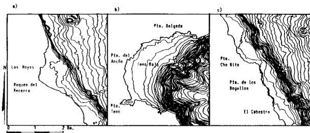
Fig. 4. Tipos de islas bajas según sus plantas. a) Triangular (Punta de San Juan, 1949, La Palma); b) En Abanico (Teno Bajo, Tenerife); c) Rectangular (Jedey-El Charco, 1585-1712, La Palma).
