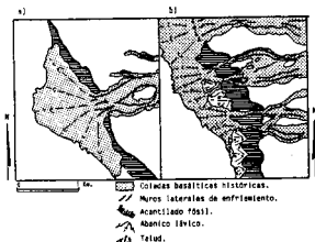
Fig. 6. Morfología de las islas bajas según los canales de derrame. a) Isla baja triangular formada a partir de una única vía de alimentación (Punta de San Juan, 1949, La Palma); b) Isla baja rectangular originada por varias vías de alimentación lávica. (Jedey, 1585, El Charco, 1712, La Palma).
