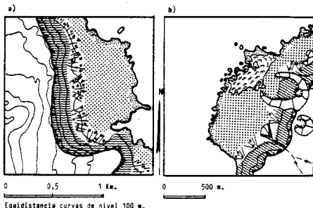
Fig. 3. Elementos de una isla baja. a) simple (Hoya del Tamaduste, El Hierro); b) compleja (Hoya del Verodal, El Hierro).
