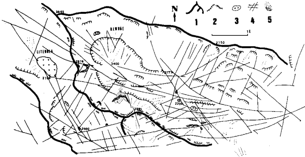
Fig. 2. Relación entre las formas de excavación glaciar, que definen el paisaje, y la red de fracturas, en Literola y Remuñe. 1: Cordales. 2: Escarpes. 3: Ibones. 4: Fracturas. 5: Depósitos.
