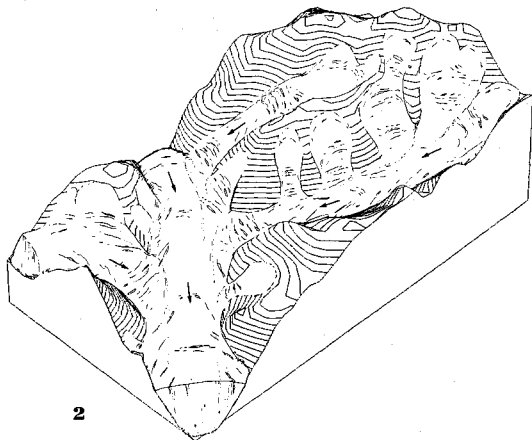
Fig. 5. 1.- Volúmenes montañosos y valles entre el Aneto (3.404 m.) y Benasque (1.138 m.). A: Aneto. B: Benasque. C: Cregüeña. ES: Valle del Esera. V: Vallibierna. E: Estós. 2.- Reconstrucción del mismo sector en el máximo glaciar pleistoceno. (Bloque por ordenador: C. Sanz Herráiz).
