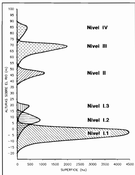
Fig. 2. Relación superficie/altura sobre el río de los niveles de terraza del Oja.
