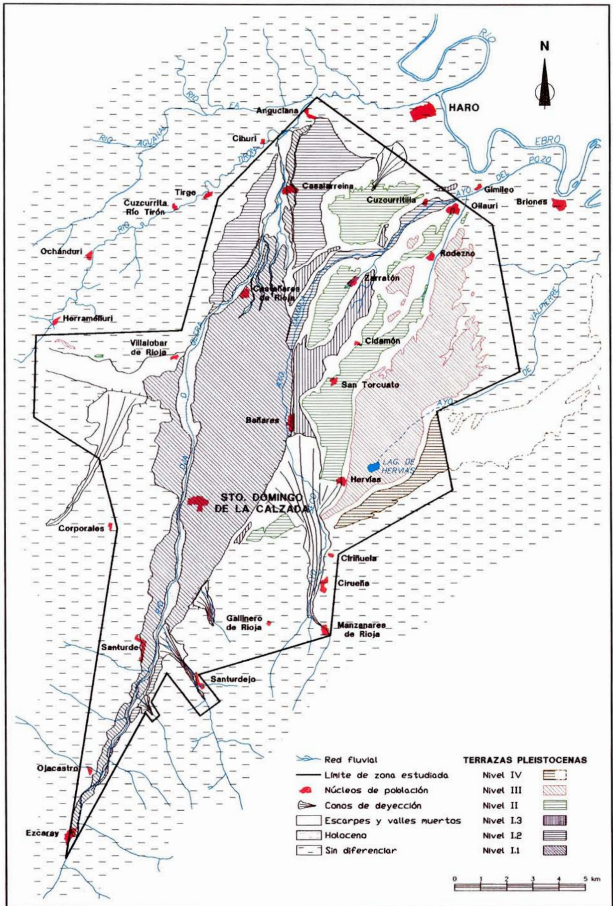
Fig. 1. Zona estudiada. Disposición de las terrazas del Oja.
