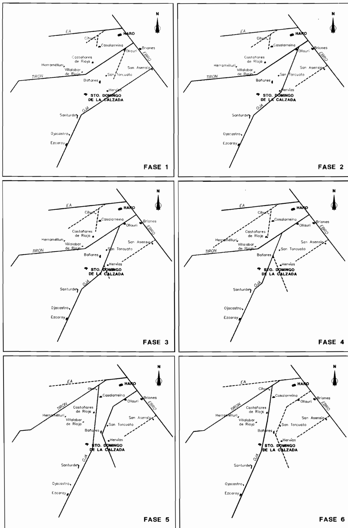
Fig. 3. Evolución de las redes fluviales de los ríos Oja y Tiron en el Pleistoceno.
