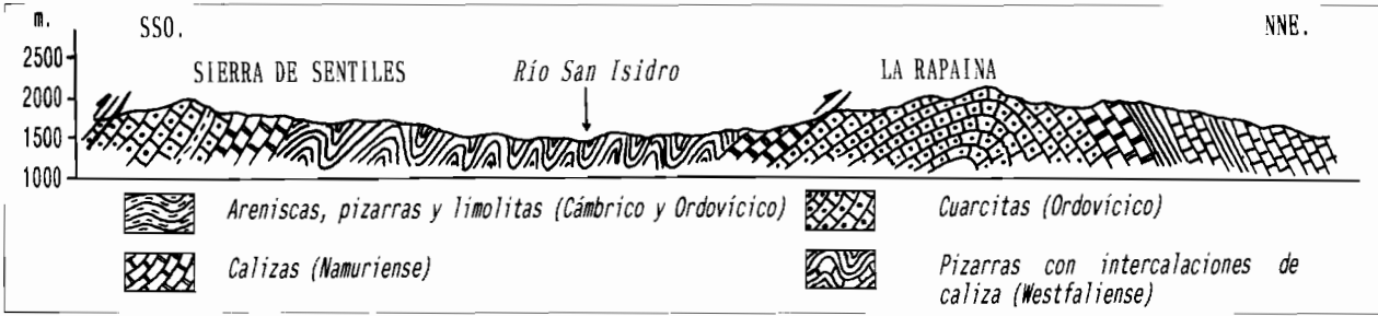
FIG. 2. Corte geológico del valle de San Isidro entre la Sierra de Sentiles y el Pico la Rapaína (escala horizontal 1:50.000).
